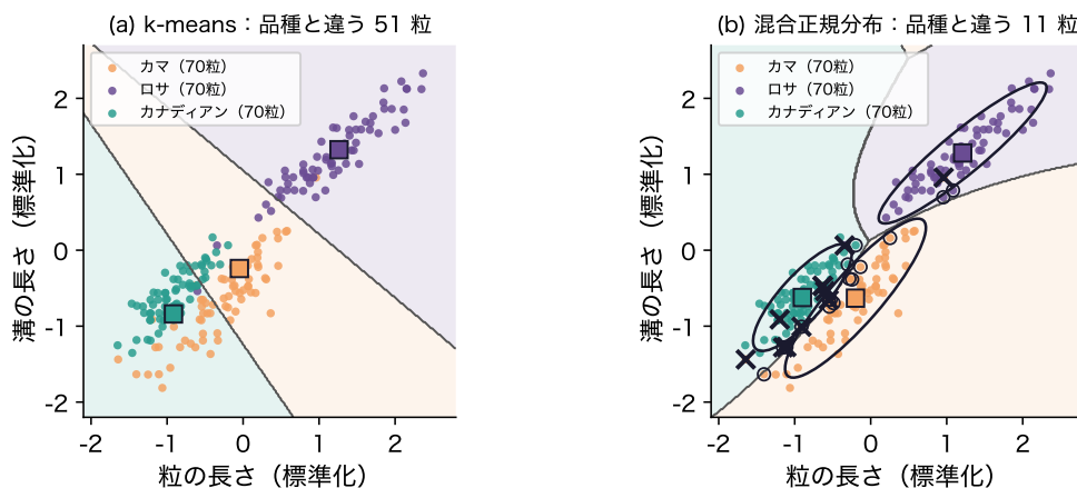
図 11: 図 10 と同じ答えの上で、粒を品種で塗り直したもの(品種は推定に使っていない)。塗り分けと灰色の線は (a) k-means、(b) 混合正規分布の境目。(b) の丸は最大の責任度が 0.9 未満の粒、× は混合正規分布の群が品種とずれた粒
