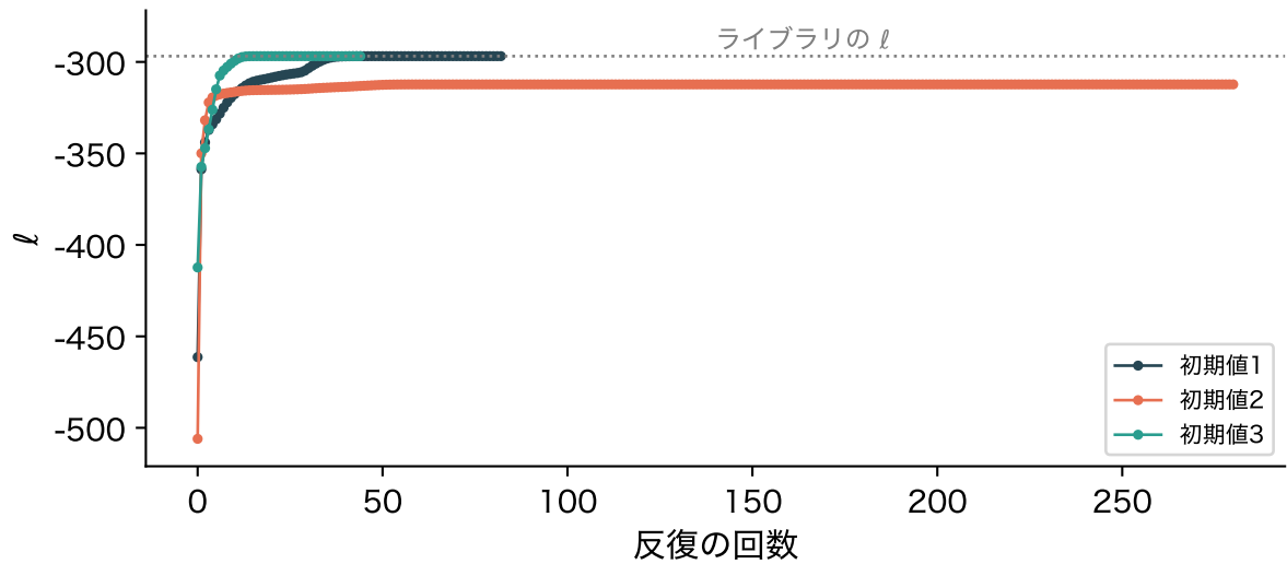
図 12: 小麦の粒の 2 列 ( k = 3 ) で、3 通りの初期値から回した EM の対数尤度 \ell の推移。点線はライブラリの \ell
