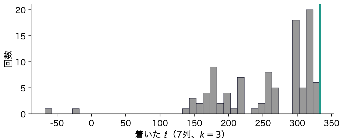
図 13: 小麦の粒の 7 列(標準化)で、群ごとの共分散を持つ EM ( k = 3 )を初期値 100 通りから回したときに着いた \ell の分布。緑の線が最大
