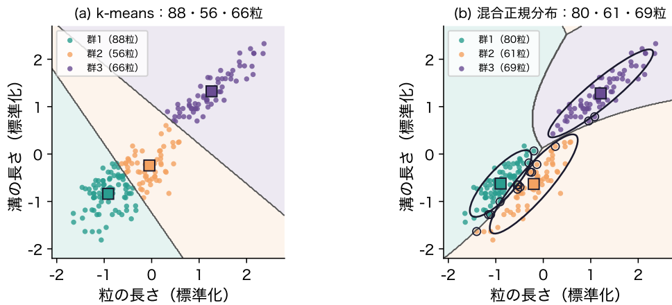
図 10: 小麦の粒の 2 列を、(a) k-means、(b) 群ごとの共分散を持つ EM で 3 つに分けたもの。■は平均、楕円は推定した \Sigma_q の形、塗り分けと灰色の線は境目、丸は最大の責任度が 0.9 未満の粒
