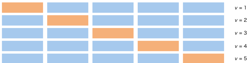
図 4: 5 分割 CV の分け方 (概念図)。各行 (行) で橙の組を測り、青の組で EM を回す
