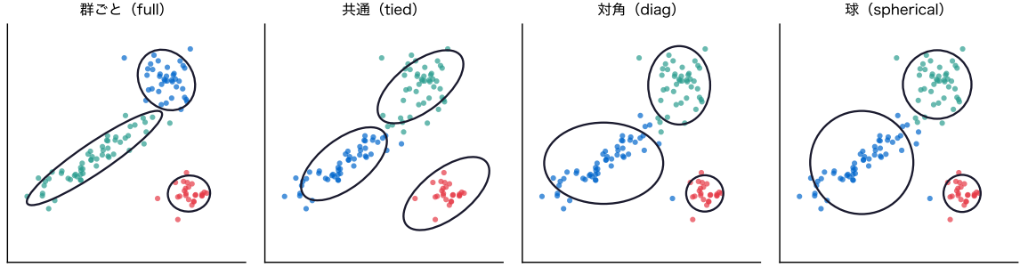
図 2: トースト 120 枚の 2 変数・3 群の人工データ(焼き時間と焼き色)に、4 つの共分散の型で k = 3 の混合正規分布を当てはめたもの。楕円は推定した \Sigma_q の形
