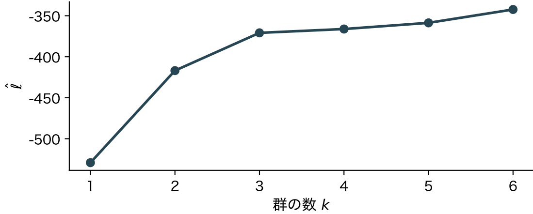
図 3: 2 変数・3 群の人工データで、群ごとの型の混合正規分布の最大の対数尤度 \hat{\ell}_k (初期値 10 通りの最良)
