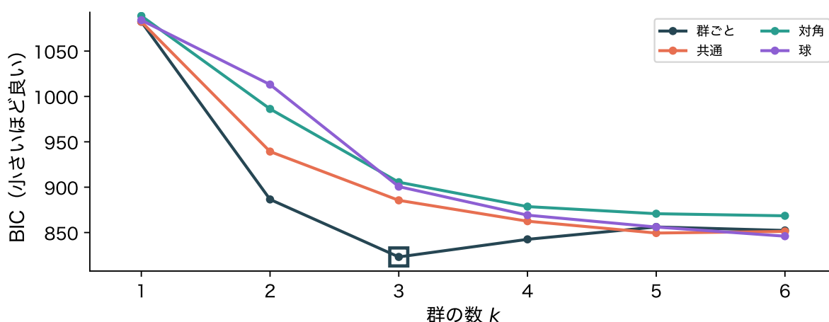
図 6: 図 5 と同じ人工データで、4 つの共分散の型の BIC を並べたもの。四角が最小
