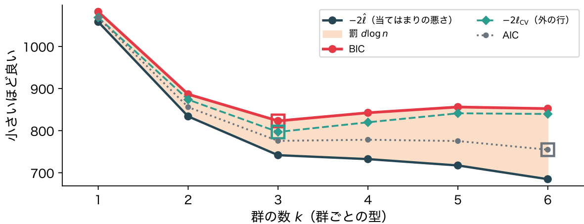
図 5: 2 変数・3 群の人工データで、群ごとの型の混合正規分布の当てはまりの悪さ -2\hat{\ell} 、BIC (橙の幅が罰 d \log n )、5 分割 CV の -2\ell_{CV} 、AIC。四角は BIC・CV・AIC が選んだ k
