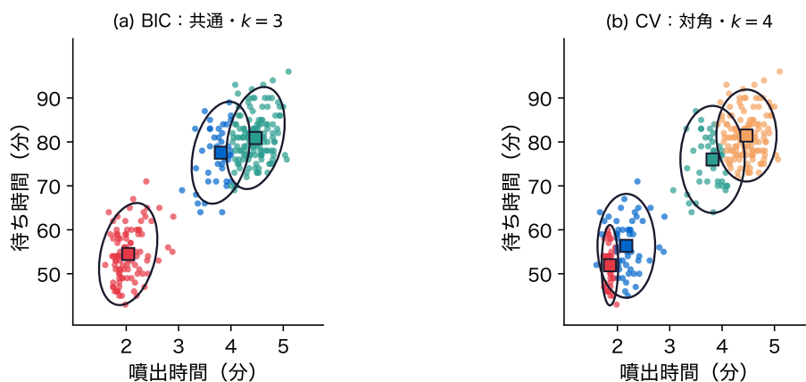
図 8: 間欠泉の 272 回の噴出で、(a) BIC、(b) 5 分割 CV が選んだ混合正規分布。色は所属(責任度が最大の群)、楕円は推定した共分散の形、■は平均
