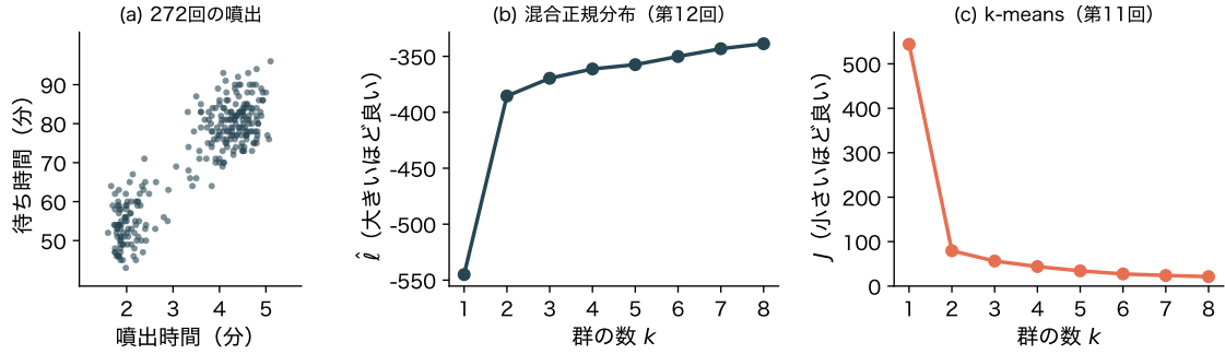
図 1: オールドフェイスフル間欠泉の 272 回の噴出。(a) 噴出時間と待ち時間(縦横は標準偏差でそろえた)、(b) 群の数 k を変えたときの混合正規分布の最大対数尤度 \hat{\ell} 、(c) k-means の目的関数 J
