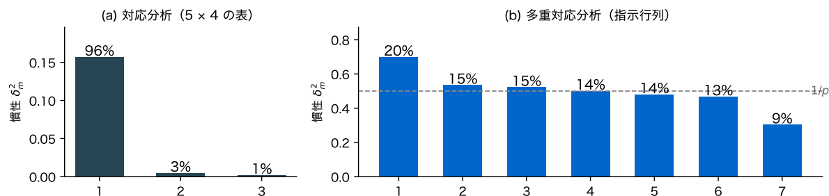
図 8: 人工の自動販売機の表の、軸ごとの慣性と寄与率。(a) 5 × 4 の表の対応分析、(b) 同じ表を 1,000 本の指示行列にした多重対応分析。破線は 1/p
