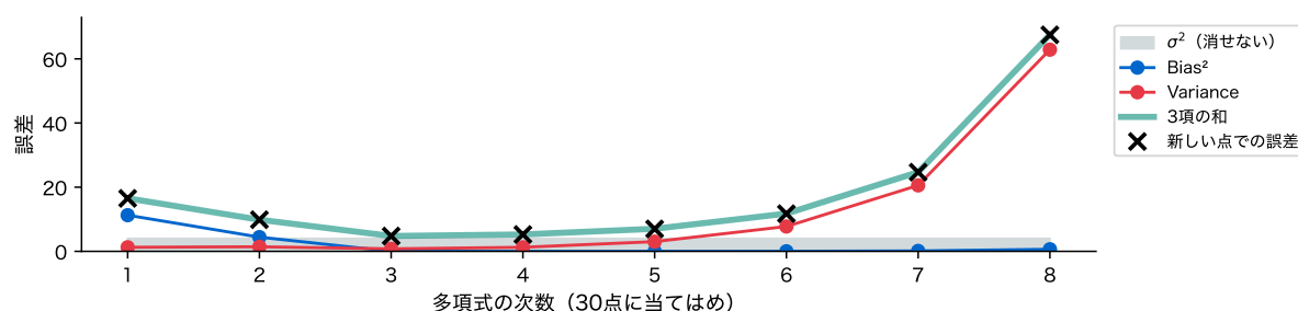
図 7: 人工データでのバイアス・バリエンス分解。30 点の訓練データを 300 回取り直して計算した 3 項と、その和(緑)、新しい点で直接測った誤差(X)
