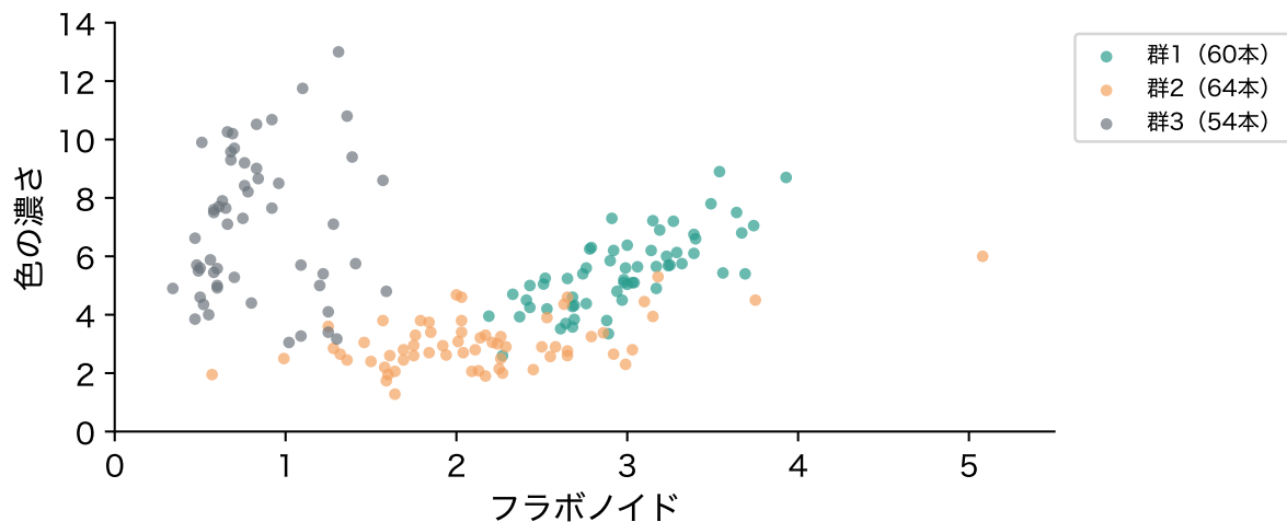
図 11: 図 1 と同じ 2 列を、13 列の k-means ( k = 3 、品種は使わない)の群で塗り分けたもの
