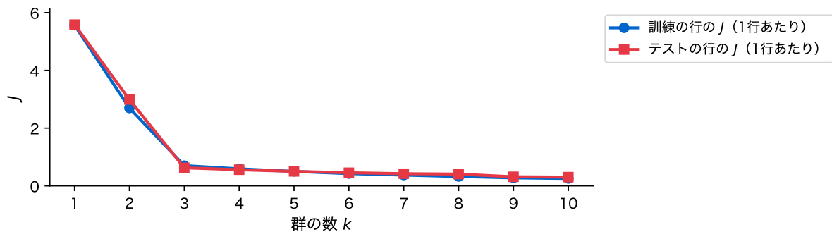
図 9: おにぎりの人工データ(訓練 200 個・テスト 100 個)での、群の数 k と 1 行あたりの J
