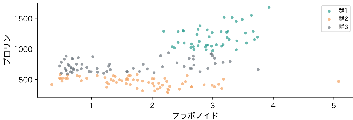
図 12: 標準化しない 13 列での k-means ( k = 3 )の群を、フラボノイドとプロリンの 2 列に塗ったもの(全 178 本)
