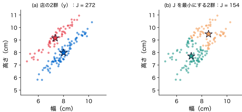
図 8: 2 つの店のおにぎり(人工データ。店の中の共分散は共通、相関 0.95)。(a) y の 2 群と各群の平均★、(b) y を使わずに J を最小にした 2 群と代表点★。 J は (b) のほうが小さい
