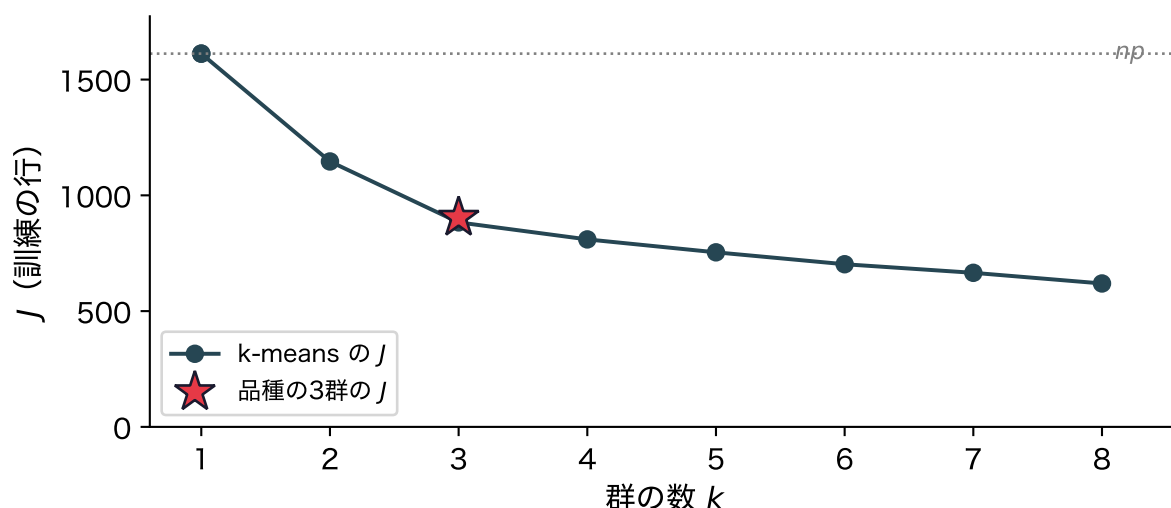
図 10: ワインのデータの訓練の行での、群の数 k と k-means の J 。点線は n \times p 。★は品種の 3 群を代表点にしたときの J
