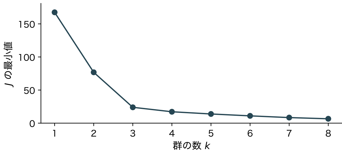
図 7: 群の数 k と J の最小値(人工データ。おにぎり 30 個)
