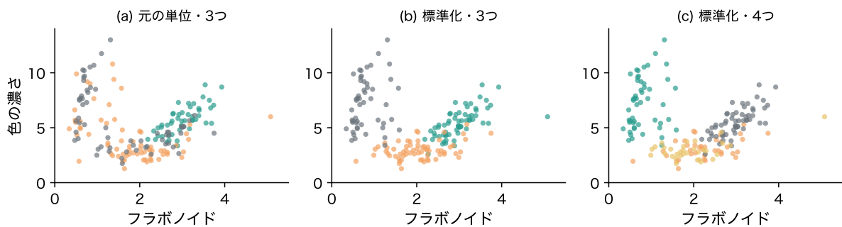
図 2: ワインの 13 列を k-means で分け、場面の 2 列に塗ったもの。(a) 元の単位のまま 3 つに、(b) 標準化してから 3 つに、(c) 標準化してから 4 つに分けた
