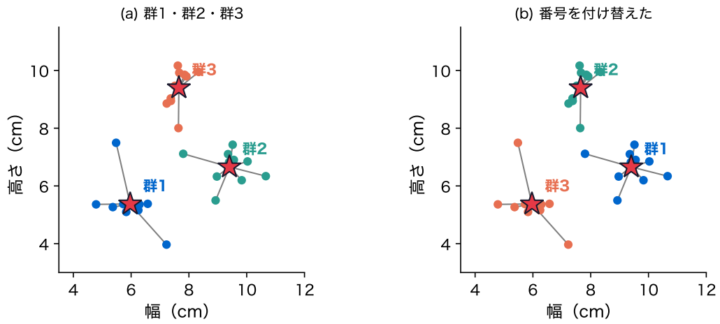
図 6: k-means の答えの番号を付け替えても J は変わらない(人工データ。おにぎり 30 個)。(a) と (b) は群の番号(と色)だけが違う
