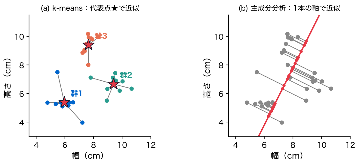
図 3: \mathbf{X} を \mathbf{X} で近似する 2 つのモデル(人工データ。おにぎり 30 個の幅と高さ)。(a) k-means (3 群)は各点を群の代表点★で、(b) 主成分分析(軸 1 本)は各点を軸に下ろした足で近似する。灰色の線が近似の誤差である
