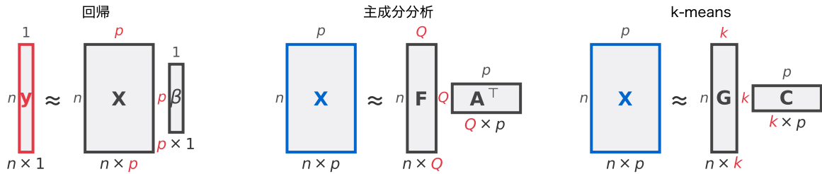
図 4: 3 つのモデルの型(概念図)。回帰は答えの列 \mathbf{y} (赤)を \mathbf{X}\boldsymbol{\beta} で、主成分分析と k-means は \mathbf{X} 自身を 2 つの行列の積で近似する
