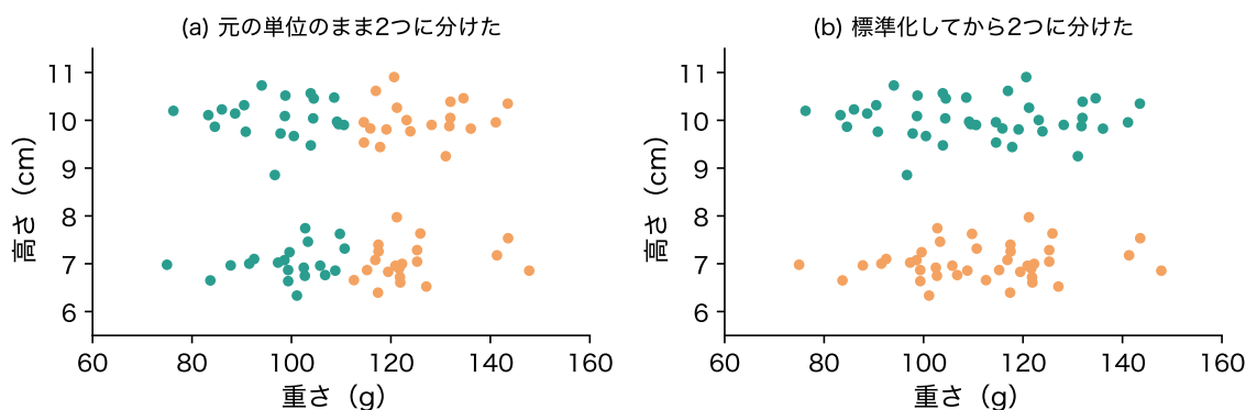
図 5: 2 つの型で握ったおにぎり 80 個(人工データ)の重さと高さを、k-means で 2 つに分けたもの。(a) 元の単位のまま、(b) 標準化してから
