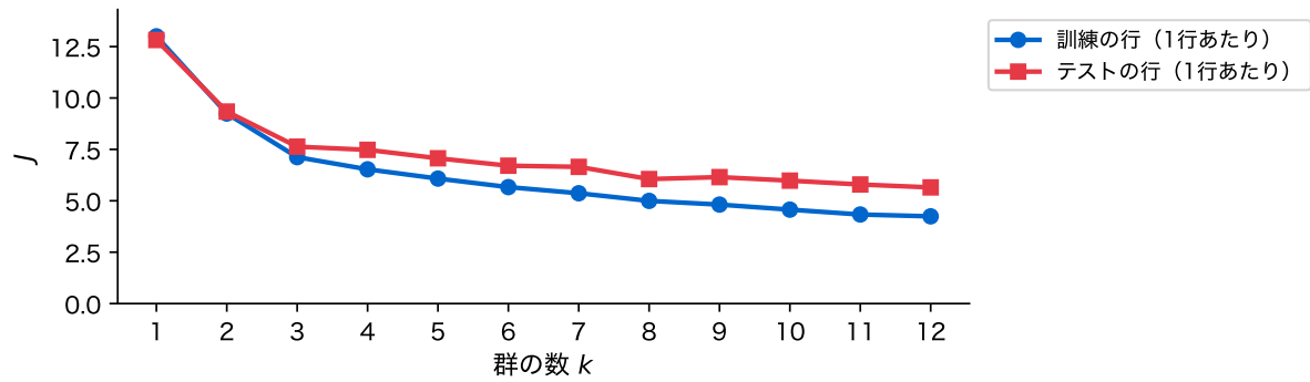
図 13: ワインのデータ(標準化した 13 列)での、群の数 k と 1 行あたりの J . 代表点は訓練の行で決めた
