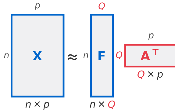
図 3: 主成分分析のモデルの型(概念図)。 n \times p の \mathbf{X} を、 n \times Q の \mathbf{F} と Q \times P の \mathbf{A}^\top の積で近似する
