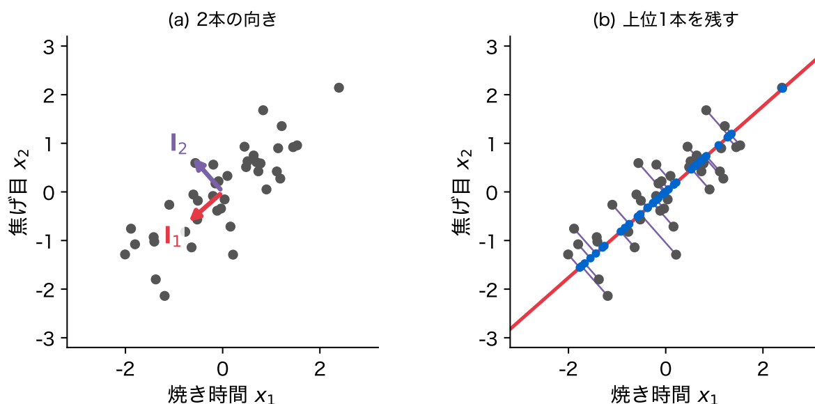
図 5: 2 列の人工データ(食パン 40 枚の焼き時間と焦げ目)の特異値分解。(a) \mathbf{L} の 2 本の向き、(b) 上位 1 本 l_1 だけを残した近似(青)と、捨てた l_2 の分の誤差(紫)
