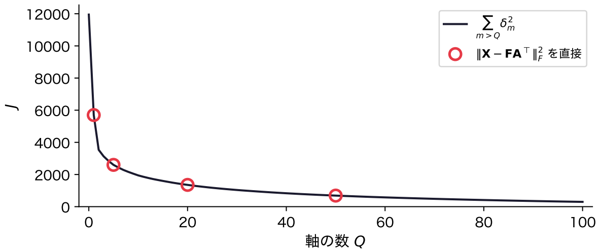
図 13: 写真の \mathbf{X} の目的関数の最小値 J = \sum_{m>Q} \delta_m^2 (線)と、近似の誤差を直接計算した値(赤い丸、 Q = 1, 5, 20, 50 )
