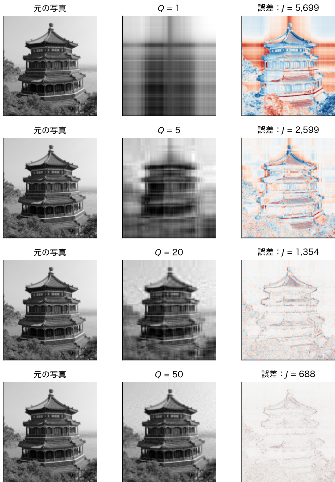
図 11: 写真の低ランク近似。各行の左から、元の写真、上位 Q 本の近似に列の平均を足したもの、誤差 \mathbf{X} - \mathbf{F}\mathbf{A}^T (赤は明るすぎ、青は暗すぎ)。上から Q = 1, 5, 20, 50
