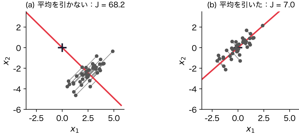
図 4: 中心化(人工データ、2 列・40 点)。(a) 点の雲を原点から離れたまま、原点を通る直線で近似したもの、(b) 列の平均を引いてから近似したもの。十字は原点
