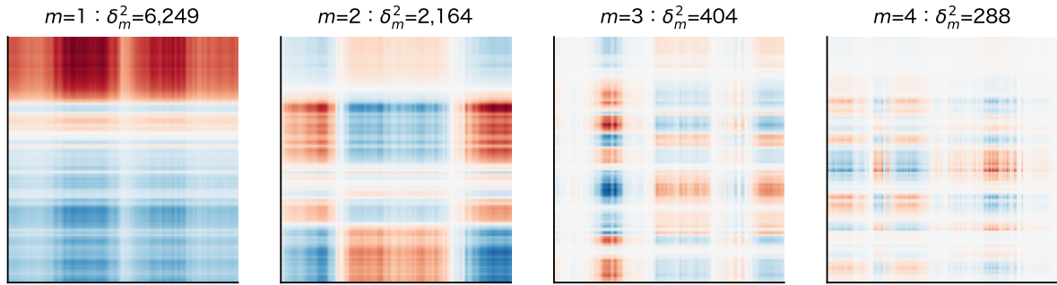
図 14: 特異値分解の 1 枚ずつの模様 \delta_m \mathbf{k}_m \mathbf{l}_m^\top (赤は正、青は負)。 m = 1 \sim 4
