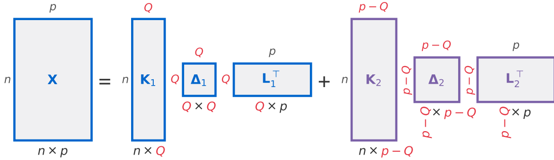
図 6: データ行列の特異値分解を、上位 Q 本(青)と残り(紫)に分けたもの。箱の縦は行の数、横は列の数。積でそろふ次元を赤で示す
