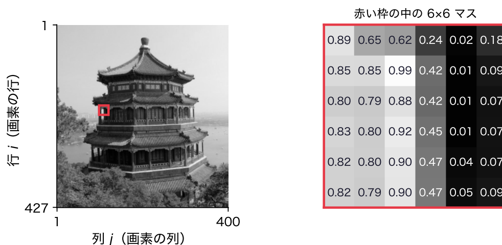
図1: (a) 写真1枚(白黒、明るさ0~1)。(b) 赤い枠の中の6×6マスの明るさ。写真は行列である
