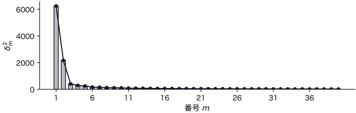
図 12: 写真の \mathbf{X} のスクリープロット(上位 40 本の \delta_m^2 )
