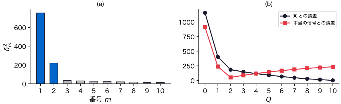
図 8: 10 台の温度計の 100 日分の人工データ(本当の信号はランク 2、そこに測りむらを足した)。(a) 特異値の二乗、(b) 残す軸の数 Q と、 \mathbf{X} との誤差 J (黒)・本当の信号との誤差(赤)
