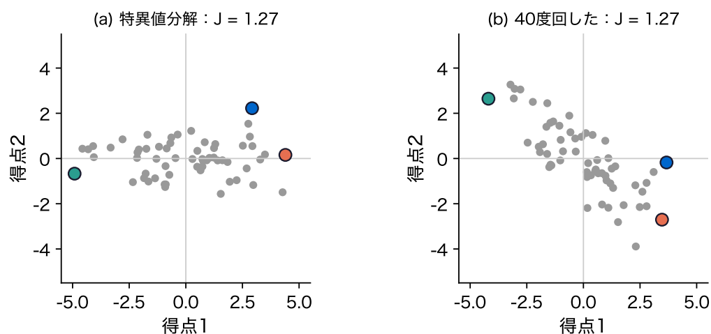
図 10: ホットケーキの人工データの得点 \mathbf{F} ( Q = 2 )。 (a) 特異値分解の答え、 (b) それを 40 度回したもの。 J は同じ。色の 3 点は同じ行
