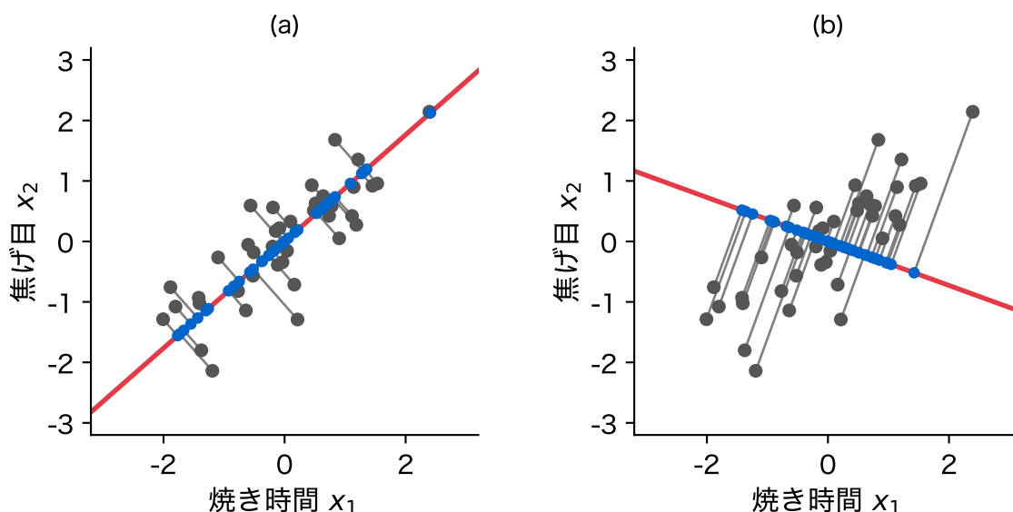
図2: 点の雲を1本の直線で近似する(人工データ、食パン40枚の焼き時間と焦げ目)。赤は長さ1の向き \mathbf{a} の直線、青は近似 f_i\mathbf{a} 、灰色は誤差。(a) 点の雲に沿った向き、(b) 160度の向き
