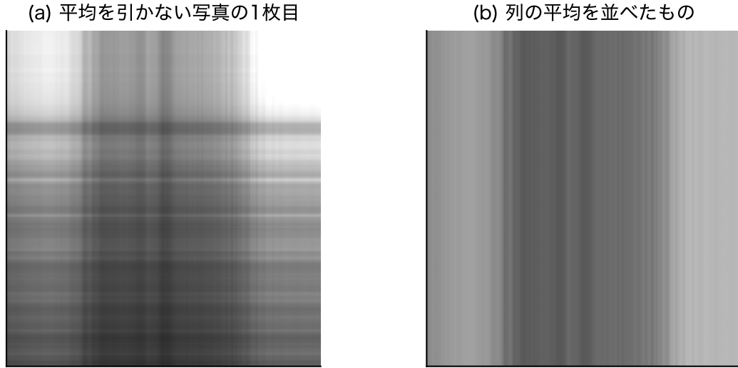
図 15: (a) 列の平均を引かない写真の 1 枚目 \delta_1 \mathbf{k}_1 \mathbf{l}_1^\top 。(b) 列の平均の明るさを各行に並べたもの
