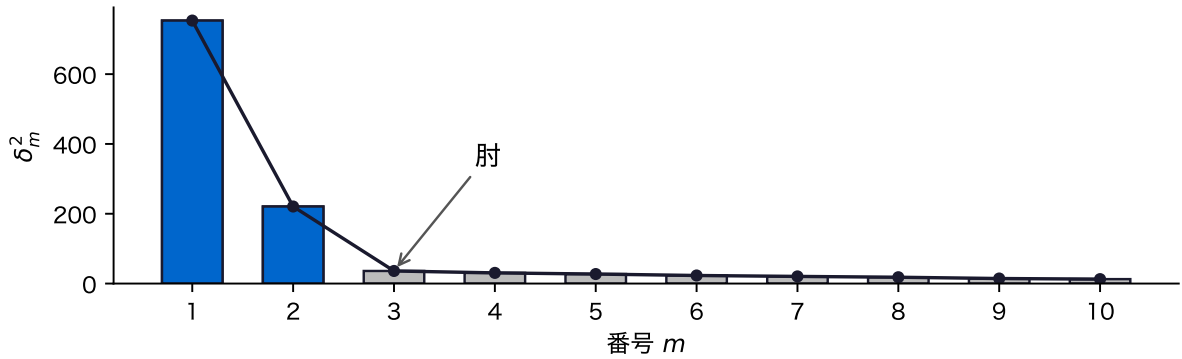
図 9: 温度計 10 台の人工データのスクリープロット。青の 2 本が肘の手前
