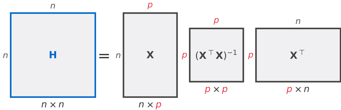
図 10: 射影行列 \mathbf{H} = \mathbf{X}(\mathbf{X}^T \mathbf{X})^{-1} \mathbf{X}^T の大きさ (概念図)。箱の縦は行の数、横は列の数。赤は掛け算でそう次元
