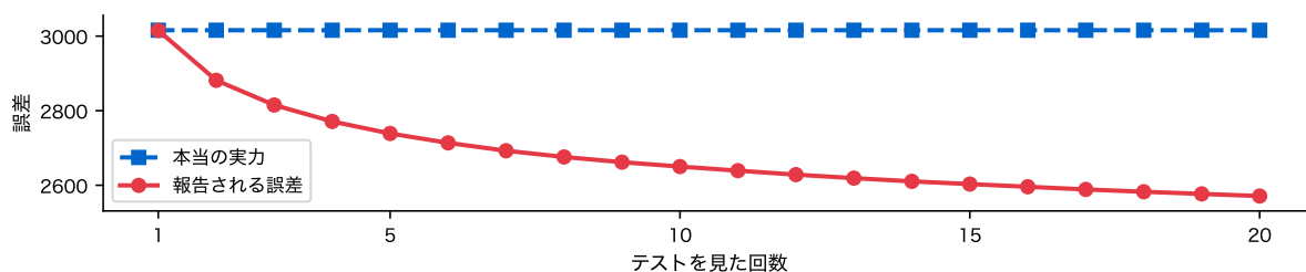
図 12: テストを見た回数と、最良の値を報告したときの誤差の期待値
