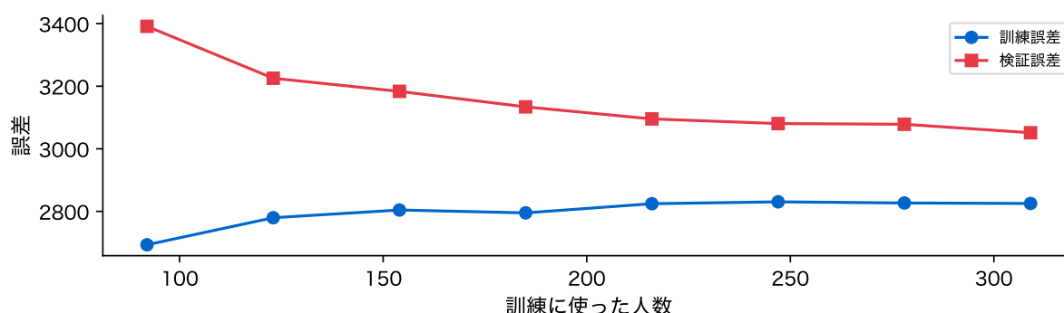
図 11: 学習曲線。訓練に使う人数を増やしたときの訓練誤差(青)と検証誤差(赤)
