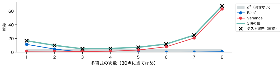
図 5: 人工データでのバイアス・バリアンズ分解。30 点の訓練データを 300 回取り直して計算した 3 項と、その和(緑)、直接測ったテスト誤差(×)
