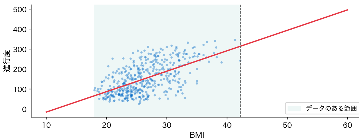
図 12: BMI だけの単回帰の直線を、データのある範囲(緑)の外まで延ばしたもの
