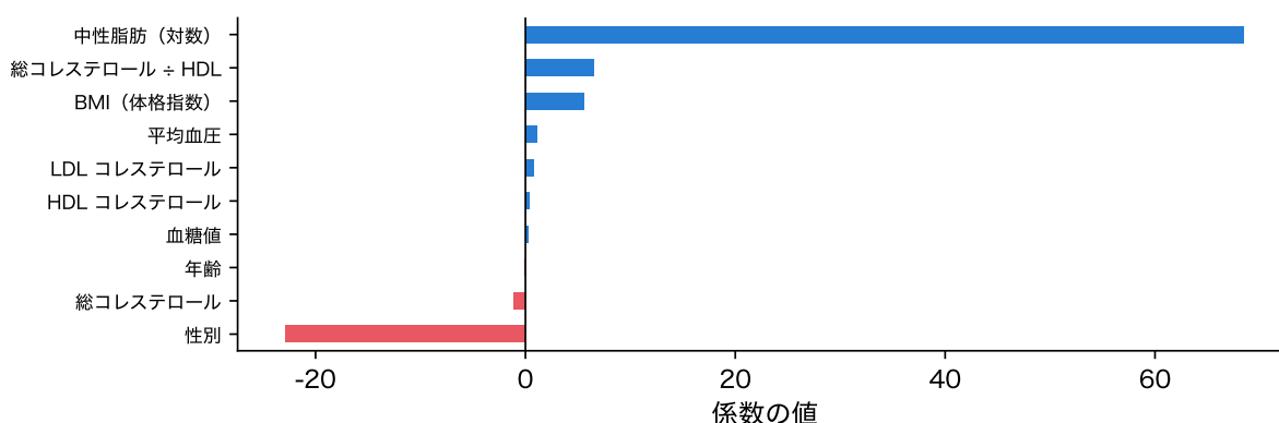
図 11: 重回帰の係数(元の単位のまま)
