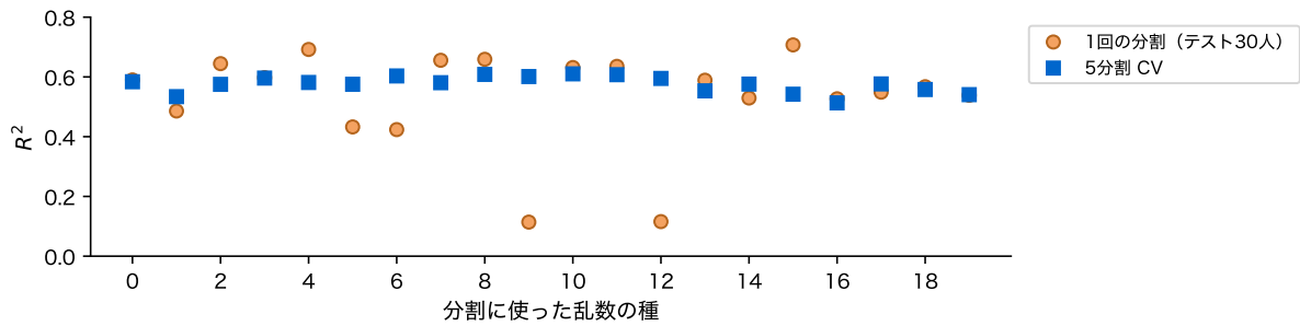
図 15: 分割の乱数を 20 通り変えたときの R^2 。1 回の分割(訓練 67 人・テスト 30 人、橙)と、5 分割 CV (青)
