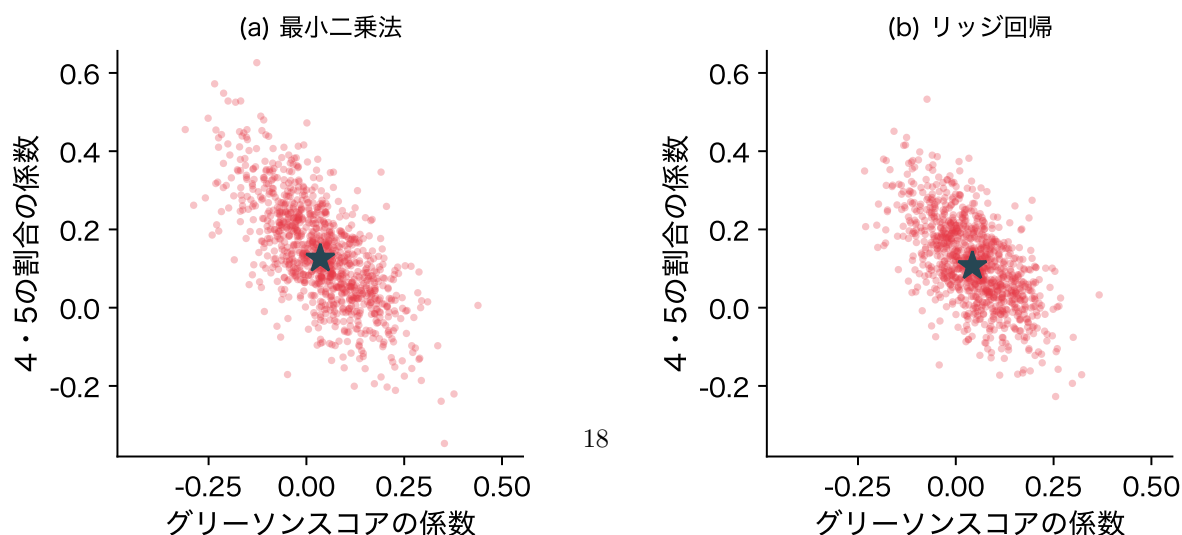
図 18: ブートストラップ 1000 回でのグリーソンスコアとグリーソン 4・5 の割合の係数(標準化した単位)。
