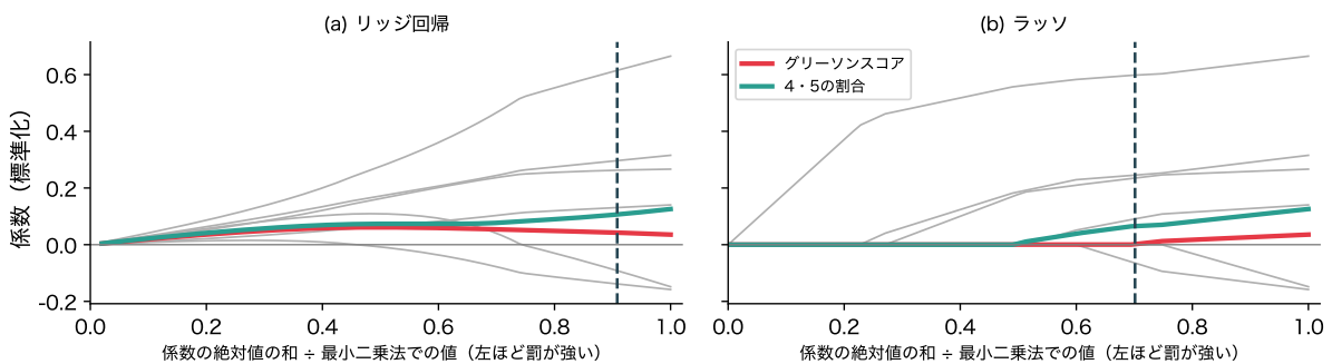
図 16: 前立腺がんのデータの係数の道筋(標準化した単位)。(a) リッジ回帰、(b) ラッソ。赤がグリーンソンスコア、緑がグリーンソン 4・5 の割合、灰はほかの 6 変数。破線は 5 分割 CV で選んだ罰の強さ
