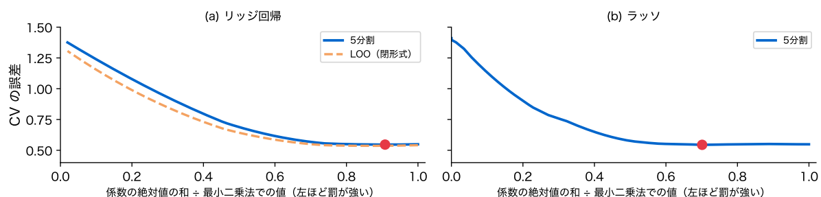
図 17: 罰の強さに対する CV の誤差(二乗平均)。(a) リッジ回帰の 5 分割(青)と LOO の閉形式(橙の破線)、(b) ラッソの 5 分割。赤は選んだ強さ
