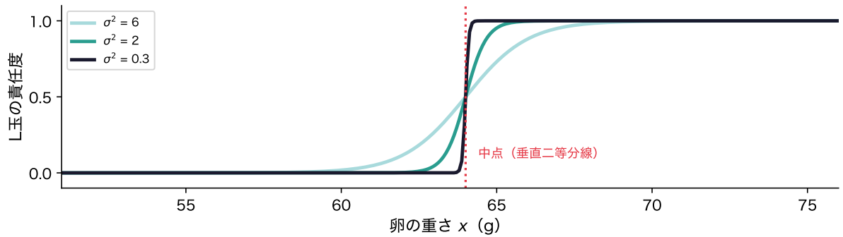
図 8: 卵の重さの 1 変数・2 群( \mu = (61, 67) 、 \pi_q は等しい)で、共通の分散 \sigma^2 ( g^2 ) を小さくしたときの L 玉の責任度(概念図)。 \sigma^2 \rightarrow 0 で中点での階段、すなわち k-means の \mathbf{G} になる
