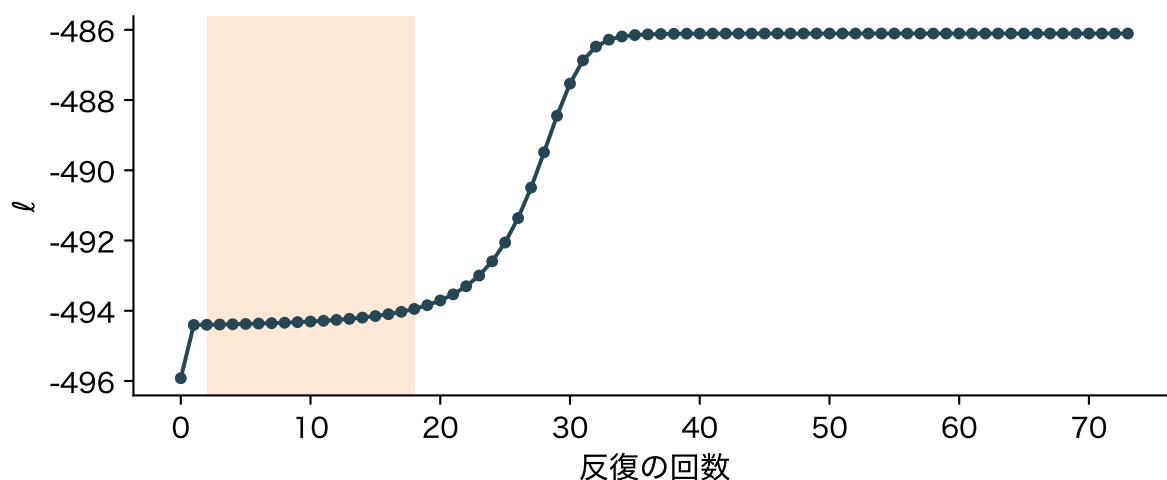
図 5: 卵 180 個の重さ(人工データ)から所属を隠し、分散を共通にした EM を回したときの対数尤度 \ell の推移。橙はほとんど動かない区間
