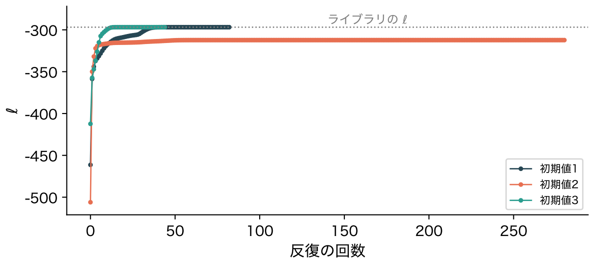
図 10: 小麦の粒の 2 列( k = 3 )で、3 通りの初期値から回した EM の対数尤度 \ell の推移。点線はライブラリの \ell
