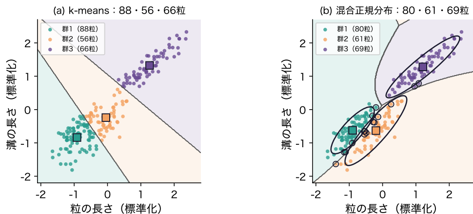
図 11: 小麦の粒の 2 列を、(a) k-means、(b) 群ごとの共分散を持つ EM で 3 つに分けたもの。■は平均、楕円は推定した \Sigma_q の形、塗り分けと灰色の線は境目、丸は最大の責任度が 0.9 未満の粒
