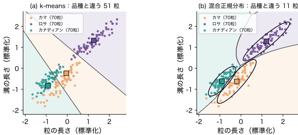
図 12: 図 11 と同じ答えの上で、粒を品種で塗り直したものの(品種は推定に使っていない)。塗り分けと灰色の線は (a) k-means、(b) 混合正規分布の境目
