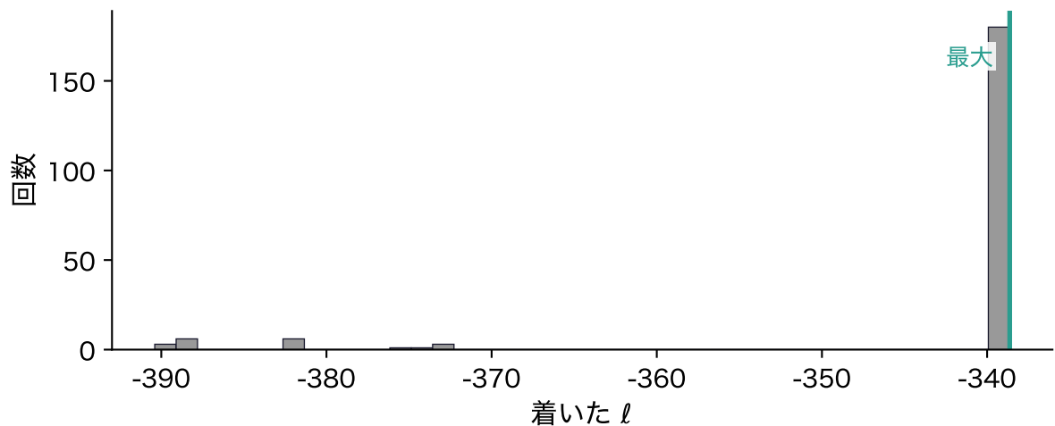
図 9: 図 7 の人工データで、初期値を変えて EM を回したときに着いた対数尤度 \ell の分布。緑の線が最大
