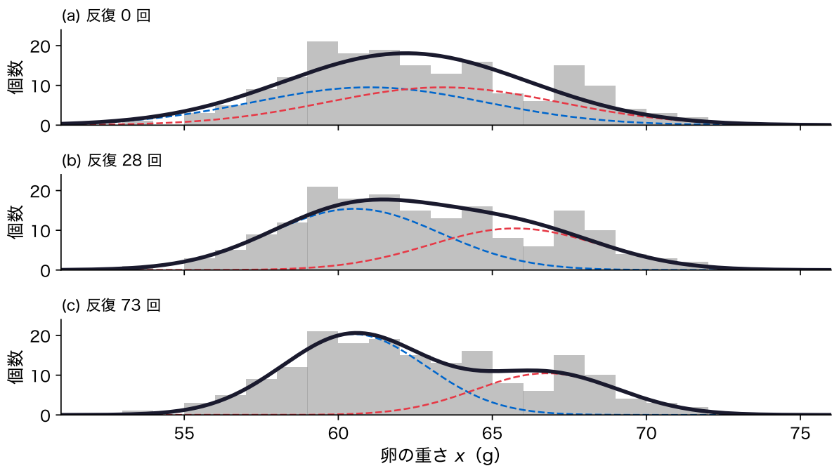
図 4: 卵 180 個の重さ(人工データ、所属は使わない)に、分散を共通にした EM を回したときの 2 つの成分(破線)と混合正規分布の密度(黒)。(a) 初期値、(b) 反復の途中、(c) 止まったとき
