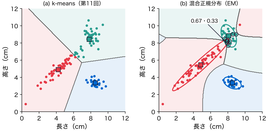
図 7: 貝殻の人工データを、(a) k-means、(b) 群ごとの共分散を持つ EM で分けたもの。色は所属((b) は責任度が最大の群)、塗り分けと灰色の線は境目、楕円は推定した \Sigma_q の形、丸は最大の責任度が 0.9 未満の点
