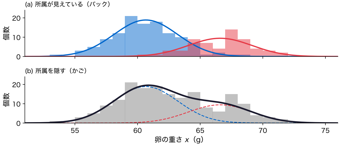
図 2: 1 変数・2 群の人工データ(卵 180 個の重さ)。(a) 所属が見えているとき(M 玉が青、L 玉が赤)、(b) 所属を隠したとき。黒は混合正規分布の密度、破線はその 2 つの成分(個数と幅 1 g に合わせて拡大した)
