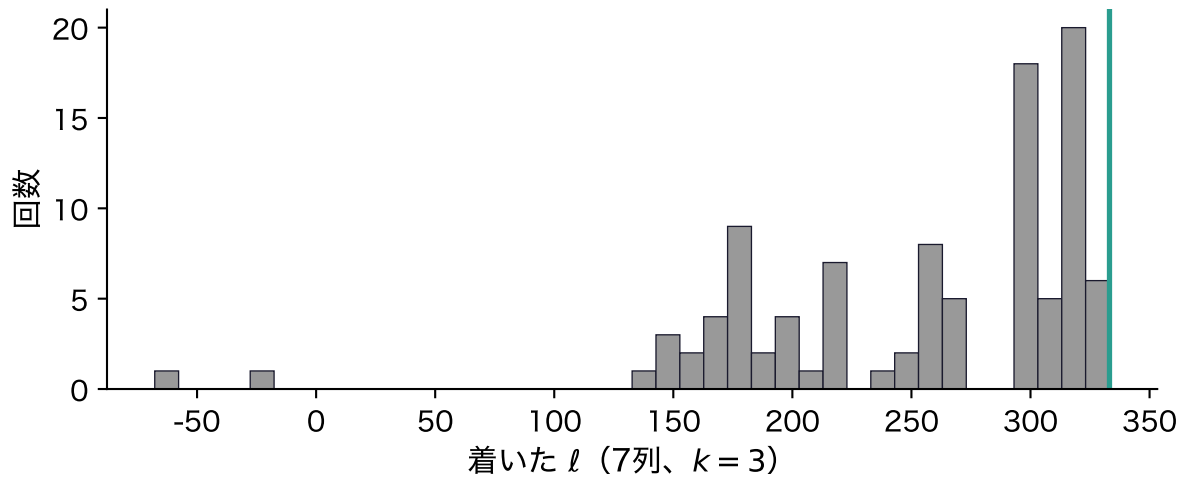
図 13: 小麦の粒の 7 列(標準化)で、群ごとの共分散を持つ EM ( k = 3 )を初期値 100 通りから回したときに着いた l の分布。緑の線が最大
