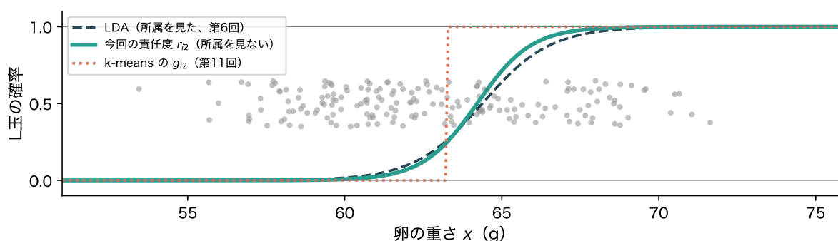
図 6: 図 2 と同じ卵の重さ(灰色の点、所属は使わない)。破線は所属を見て推定した LDA の事後確率、緑は EM で求めた L 玉の責任度、点線は k-means の所属
