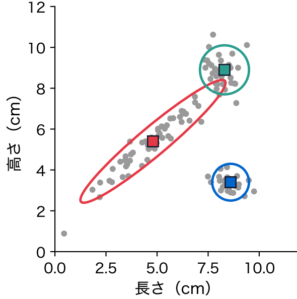
図 3: 2 変数・3 群の人工データ(貝殻の長さと高さ。赤がハマグリ、青がマテガイ、緑がホタテ)。楕円は、データを作った 3 つの正規分布の (\tilde{\mathbf{x}} - \boldsymbol{\mu}_q)^\top \boldsymbol{\Sigma}_q^{-1}(\tilde{\mathbf{x}} - \boldsymbol{\mu}_q) = 4 の線、■はその平均
