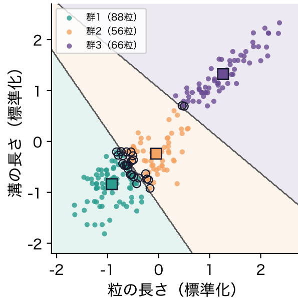
図 1: 小麦の粒 210 粒の粒の長さ(標準化)と溝の長さ(標準化)を k-means ( k = 3 )で分けた答え。■は代表点、灰色の線が境目(垂直二等分線)、丸は境目のすぐそばの粒
