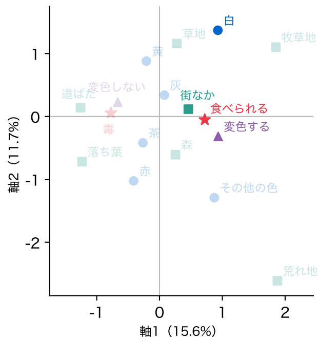
図 13: 多重対応分析の地図で、食べられる・街なか・白・傷で変色するだけを濃く描いたもの
