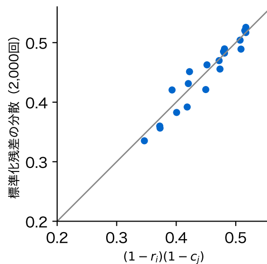
図 9: 食べられるか × かさの色の表と同じ周辺の独立のモデルから作った 2,000 表での、標準化残差の分散。横軸は (1 - r_i)(1 - c_j) 、線は y = x
