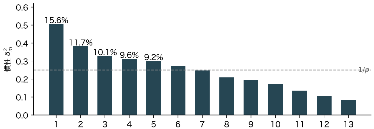
図 12: 食べられるか・かさの色・生える場所・傷で色が変わるかの多重対応分析の、軸ごとの慣性。破線は 1/p
