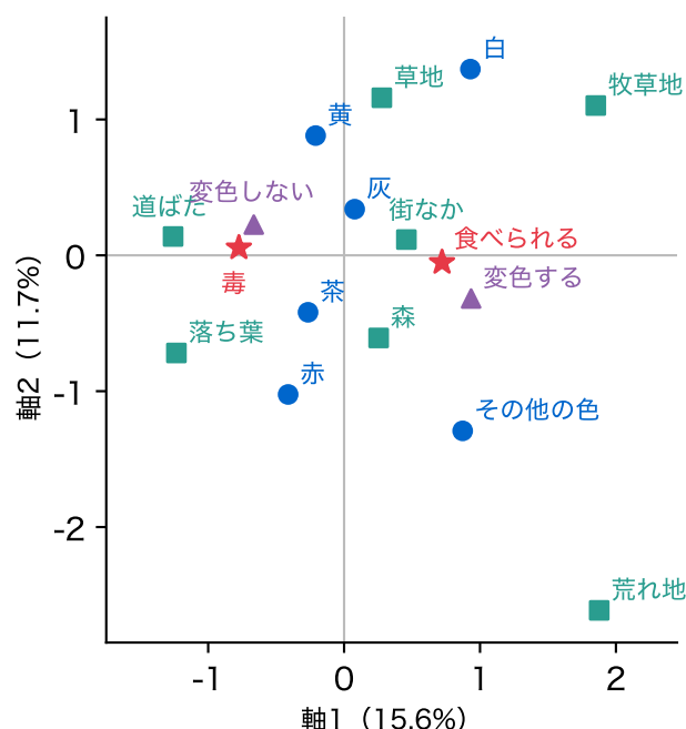
図 11: 食べられるか・かさの色・生える場所・傷で色が変わるかの多重対応分析の地図。赤の星が食べられるか、青の丸がかさの色、緑の四角が生える場所、紫の三角が傷
