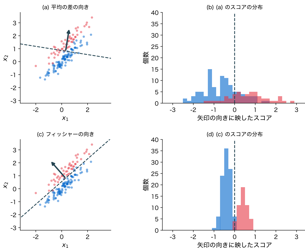
図 3: 2 変数・2 群の人工データ ( y = 0 が青、 y = 1 が赤)。(a)(b) 平均の差の向き \mathbf{d} に映したとき、(c)(d) フィッシャーの向き \mathbf{S}_W^{-1} \mathbf{d} に映したとき。矢印が向き、破線が midpoint を通る境界。(b)(d) は映したスコアの分布
