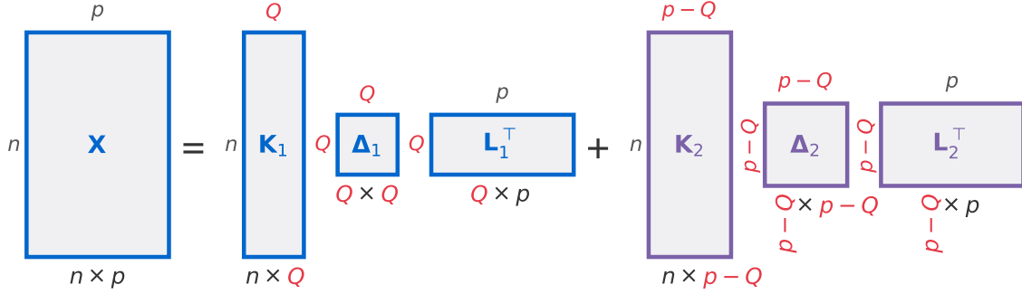
図 3: データ行列の特異値分解を、上位 Q 本(青)と残り(紫)に分けたもの。箱の縦は行の数、横は列の数。積でそろ次元を赤で示す
