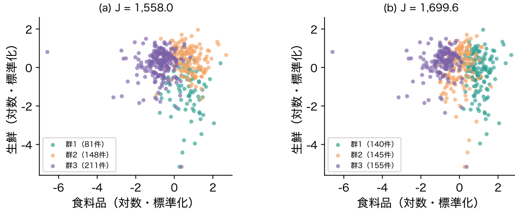
図 16: 卸売の顧客を k = 3 に分けた 2 つの答え。(a) 100 通りのうち J が最小、(b) J が最大。群の番号は食料品の購入額の中央値が大きい順
