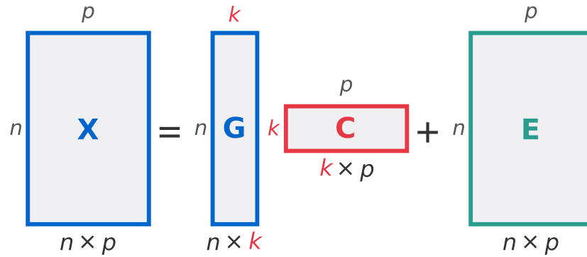
図 3: k-means のモデルの型(概念図)。 n \times p の \mathbf{X} を、 n \times k の \mathbf{G} と k \times p の \mathbf{C} の積と誤差 \mathbf{E} に分ける
