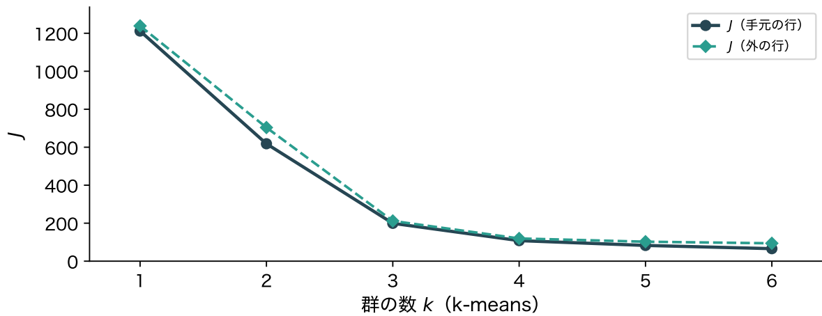
図 7: 図 5 と同じ人工データで、k-means の J を手元の行(全行で当てはめ)と外の行(5 分割)で測ったもの
