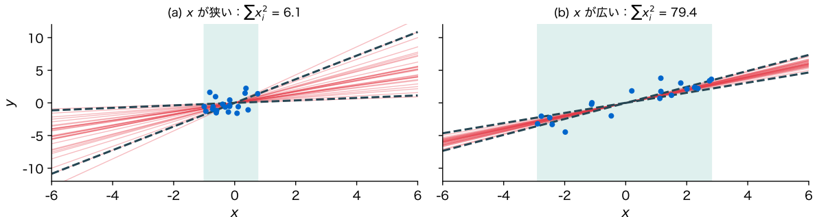
図 6: 人工データで、 x を固定したまま y を 30 回取り直して引いた原点を通る直線(赤)。(a) x が狭い範囲、(b) 広い範囲。青は 1 回ぶんの点、緑はデータのある範囲、破線は予測の \pm 2 標準偏差(後述)
