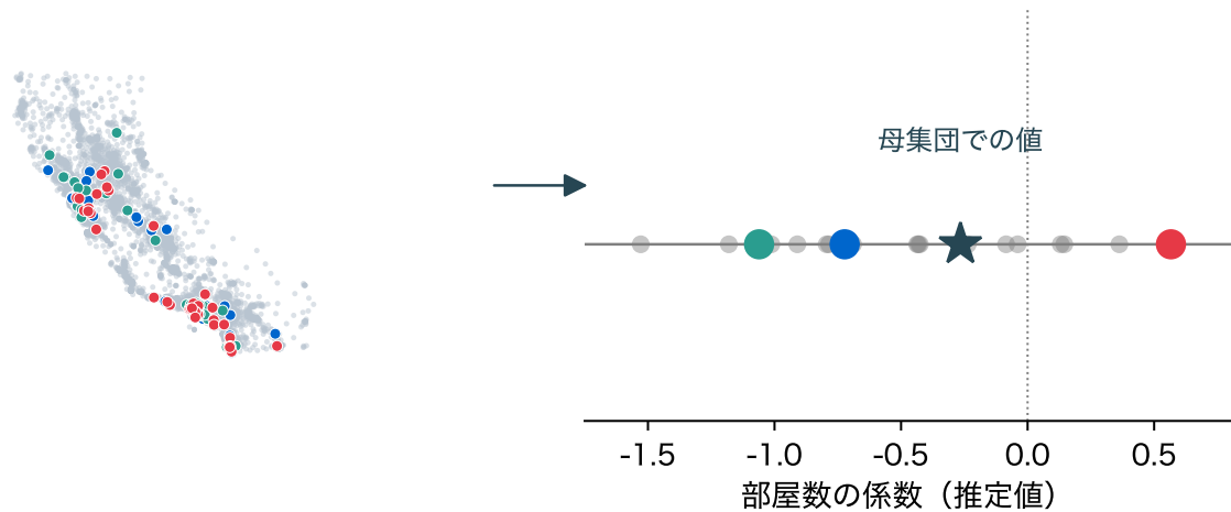
図 23: 20,640 地区を母集団とみなしたときの、40 地区の標本 3 つ(左、青・緑・赤)と、標本ごとの部屋数の係数の推定値(右、灰色は 20 回ぶん)。★は全地区での値、0 より右は符号が逆
