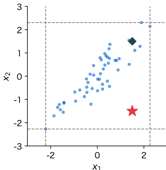
図 16: 相関 0.9 の 2 列(人工データ、50 行)。破線は各列の最小値と最大値。★はどちらの列も範囲の中だが雲の外点、◆は原点から同じ遠さで雲に沿った点
