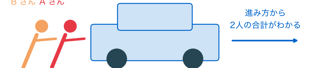
図 7: 共線性のたとえ(概念図)。いつも 2 人で押す車では、進み方から 2 人の力の合計はわかるが、内訳はわからない
