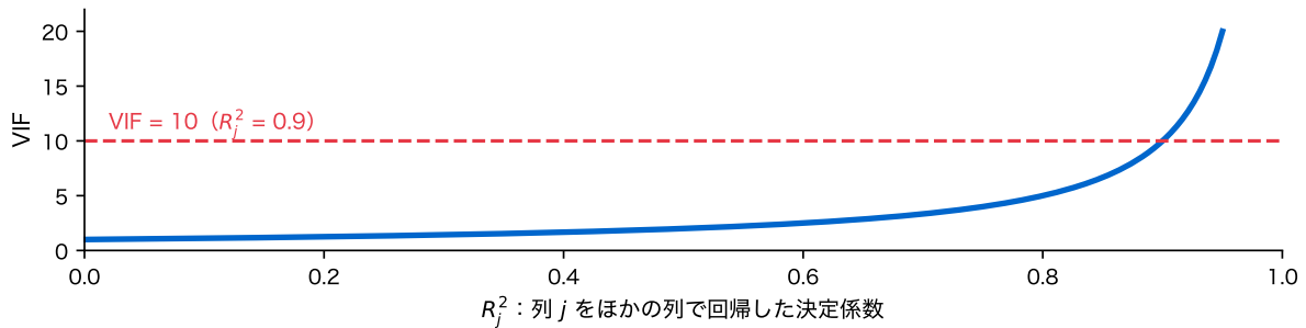
図 9: 分散拡大係数 VIF_j = 1/(1 - R_j^2) と、目安とされる VIF = 10 (赤の破線)
