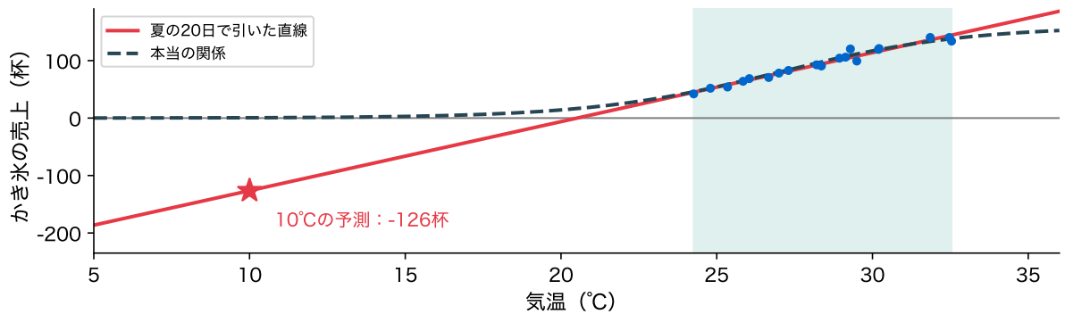
図 13: かき氷の売上と気温(人工データ)。緑は記録のある範囲、赤は記録から引いた直線、破線は本当の関係。 ★は記録がない 10 °C の日の予測
