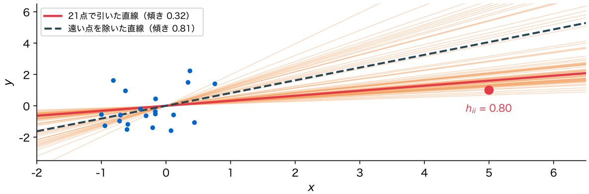
図 12: てこ比の大きい 1 点(人工データ)。青の 20 点に x = 5 の赤の点を足した。赤の実線は 21 点で、黒の破線は赤の点を除いて引いた直線。橙は 21 行を復元抽出して引き直した直線(80 回ぶん)
