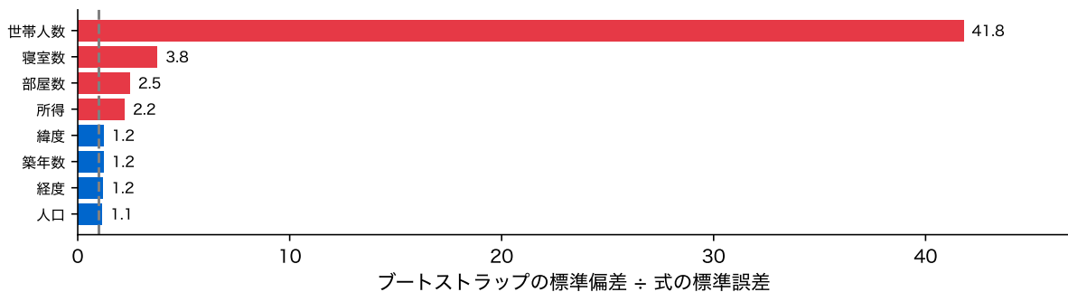
図 21: 地区を復元抽出して 1000 回当てはめ直したときの係数の標準偏差を、式の標準誤差で割った比。破線は 1 (式どおり)
