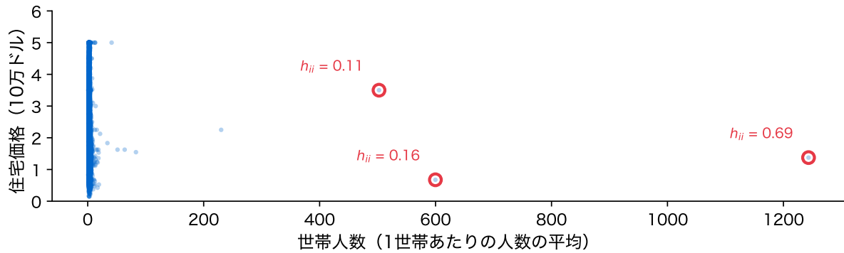
図 22: 世帯人数と住宅価格。赤丸は世帯人数の大きい 3 地区で、数字はそのてこ比
