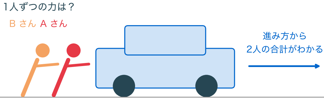
図 6: 共線性のたとえ(概念図)。いつも 2 人で押す車では、進み方から 2 人の力の合計はわかるが、内訳はわからない
