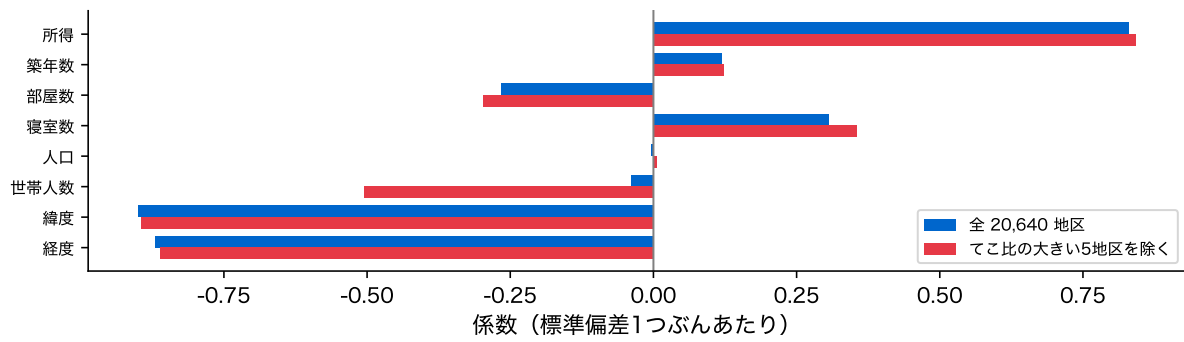
図 23: 全地区で当てはめた係数(青)と、てこ比の大きい 5 地区を除いて当てはめた係数(赤)。標準偏差 1 つぶんあたり
