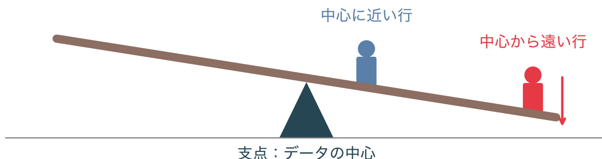
図 11: てこ比のたとえ(概念図)。直線はデータの中心を支点に回る板で、中心から遠い行ほど板を大きく傾ける
