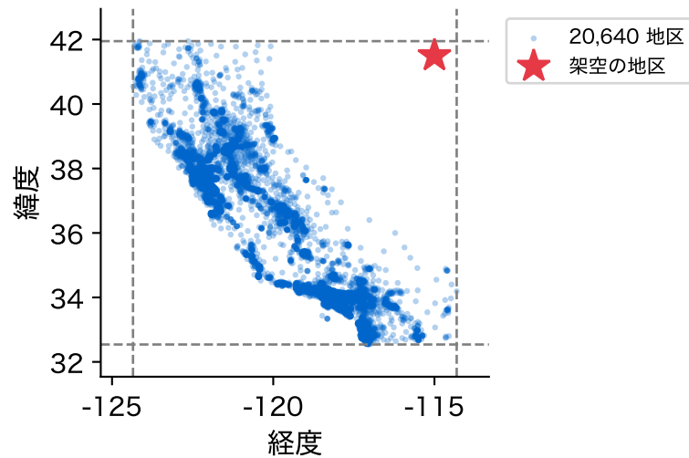
図 24: 地区の緯度と経度と、架空の地区(★)。破線は緯度・経度それぞれの最小値と最大値
