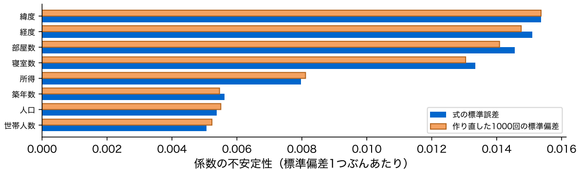
図 18: 係数の不安定性。式 \hat{\sigma}^2(\mathbf{X}^\top \mathbf{X})^{-1} による標準誤差(青)と、 \mathbf{X} を固定して目的変数を 1000 回作り直したときの標準偏差(橙)。標準偏差 1 つぶんあたりに直してある
