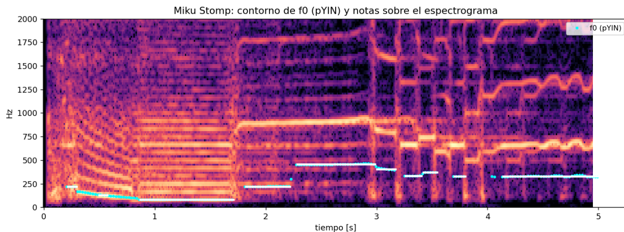
Fig. 8. Miku Stomp: contorno de f0 (pYIN) y notas detectadas sobre el espectrograma de la guitarra (tras estabilizar el seguimiento).
