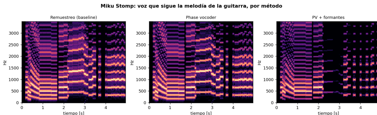
Fig. 9. Miku Stomp: voz que sigue la melodía de la guitarra, sintetizada con cada método de pitch-shift.
