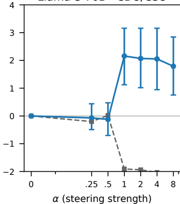
Llama-3 70B · CDU/CSU
