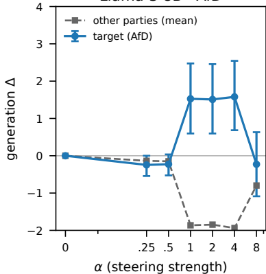
Llama-3 8B · AfD
