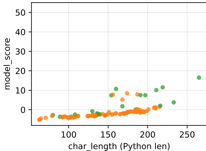
v1 / sentseq-3e4
