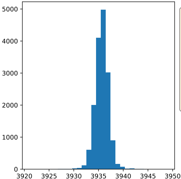
encoder-data-1 (ERCK-0505-360)
