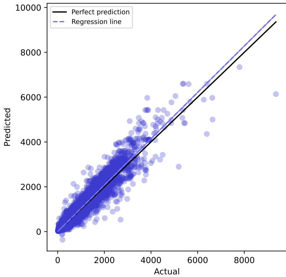
CatBoost
