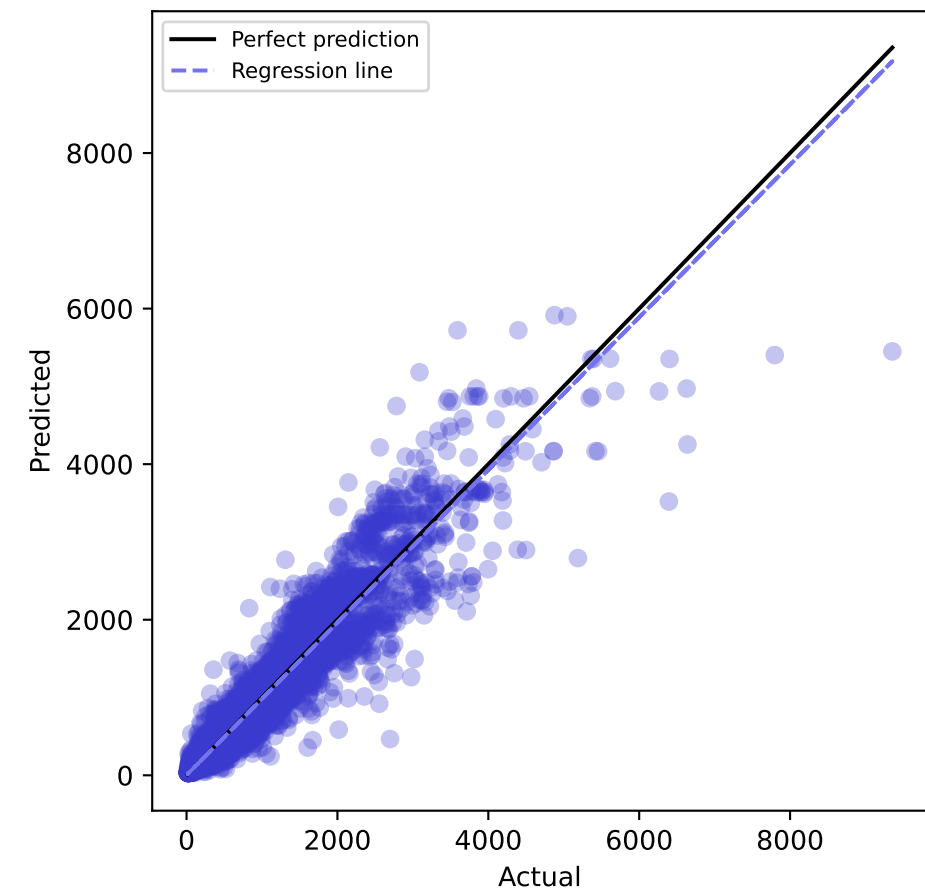
CatBoost
