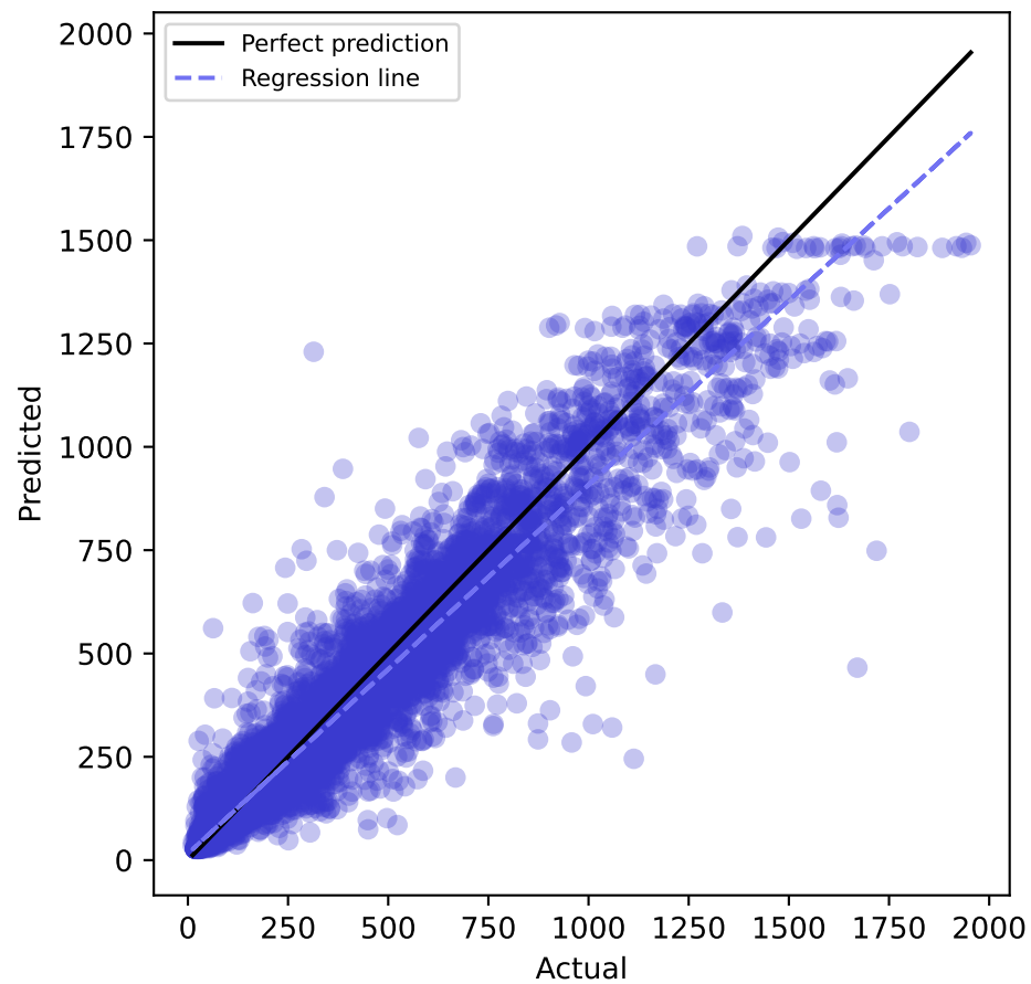
CatBoost
