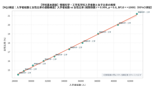
図2 情報科学・工学系学科入学者数と女子比率の推移の相関構造および比較分析（95%CI併記）
