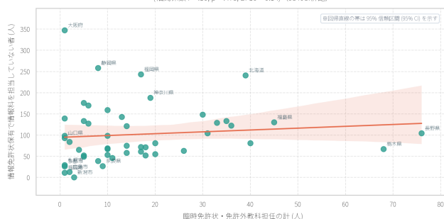
図2 臨時免許状・免許外教科担任の計と情報免許状保有で情報科を担当していない者の関連（回帰直線と95%信頼区間の帯）
