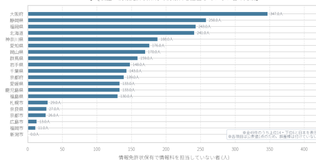
図1 情報免許状保有で情報科を担当していない者の値の比較（上位・下位と日本を抜粋）
