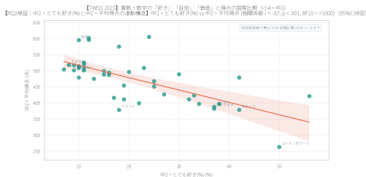
図2 算数・数学の「好き」「自信」「価値」と得点の国際…の関連構造および比較分析 (95%CI併記)
