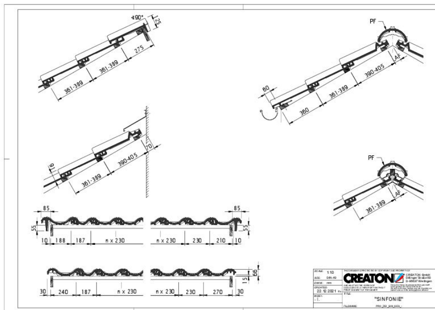
Zeichnung SINFONIE Gesamtansicht GES
