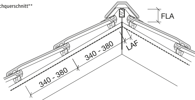
Dachquerschnitt**
