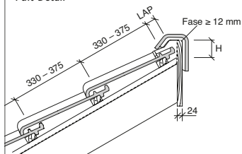
Ortgang - Detail mit Doppelwulstziegel*/**
