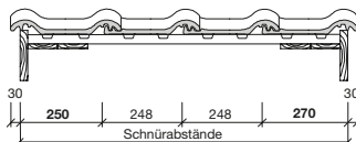
Ortgang - Detail mit Doppelwulstziegel*/**
