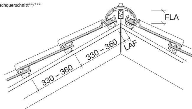
Dachquerschnitt**/***
