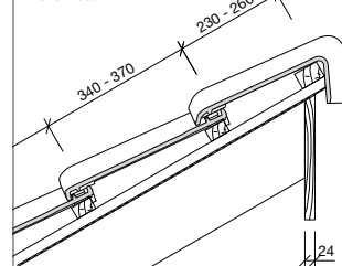
Pult-Detail**
