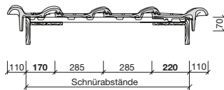
Ortgang - Detail mit Ortgangziegel*/**
