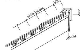
Pult-Detail**
