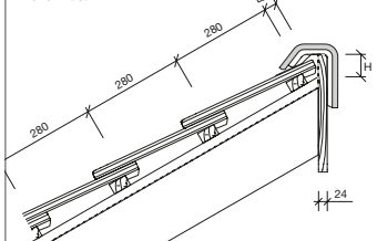
Pult-Detail**
