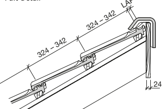
Pult-Detail**
