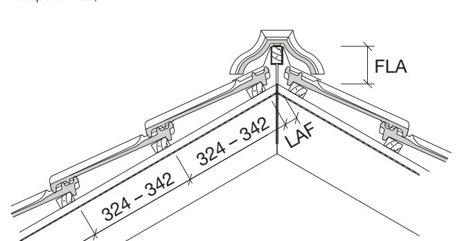
Dachquerschnitt**/***
