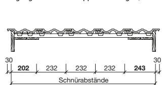
Ortgang - Detail mit Doppelwulstziegel*/**
