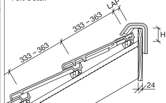
Pult-Detail**
