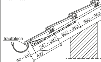
Trauf-Detail**
