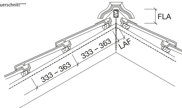
Dachquerschnitt***
