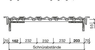
Ortgang - Detail mit Ortgangziegel*/**
