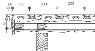
Ortgang - Detail mit Ortgangziegel**
