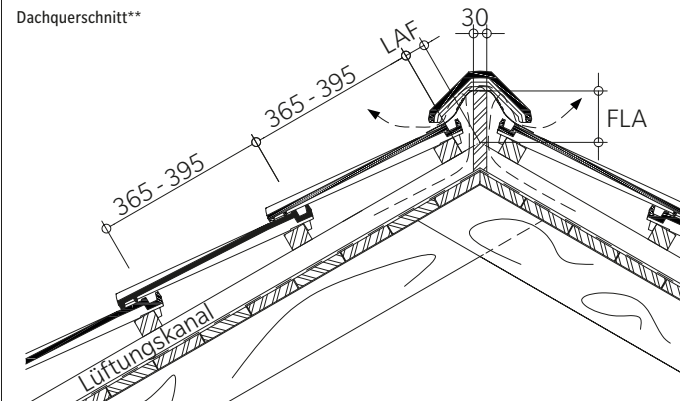
Dachquerschnitt**
