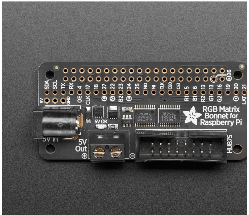
Adafruit RGB Matrix Bonnet — lato componenti
