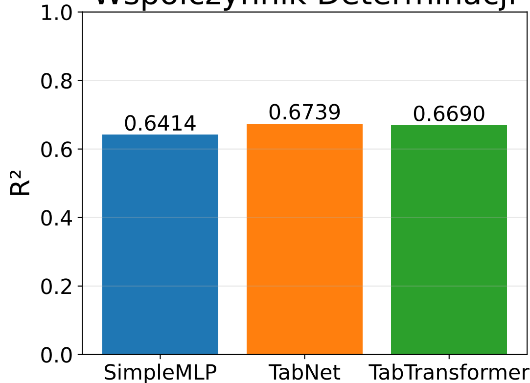
Współczynnik Determinacji
