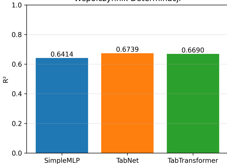
Współczynnik Determinacji
