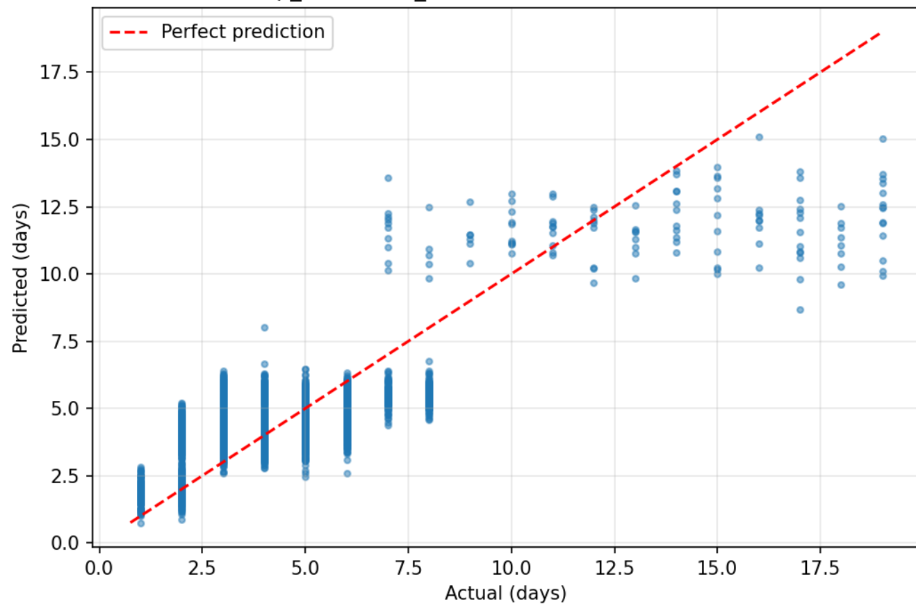
mlp_20251216_221732 - Predictions vs Actual
