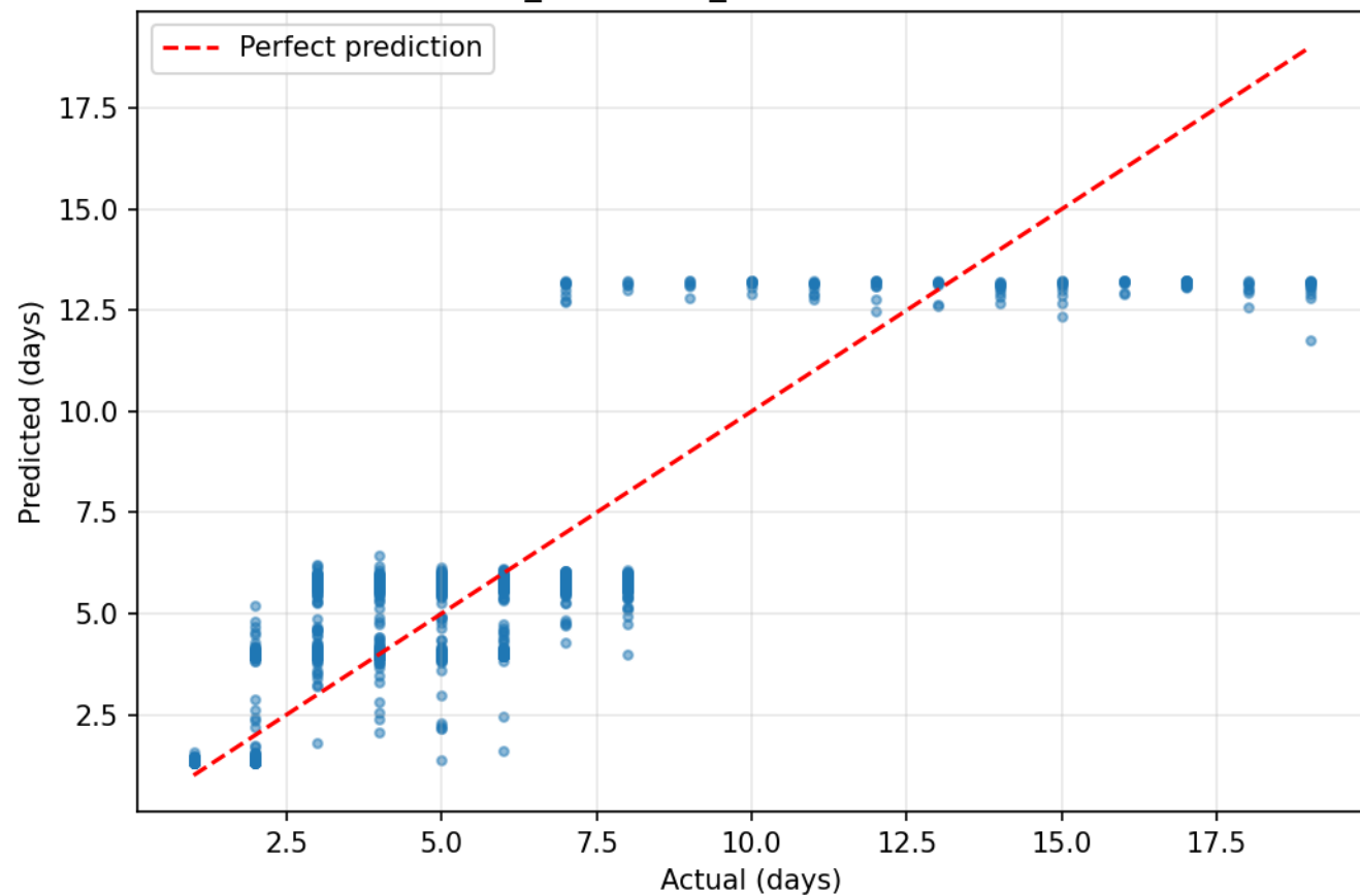
tabtransformer_20251217_101214 - Predictions vs Actual
