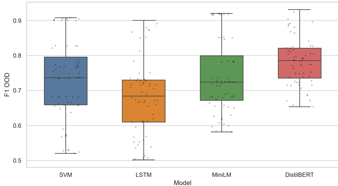
Rozkład F1 OOD (60 pomiarów per model: 4 train \times 3 OOD \times 5 fold)
