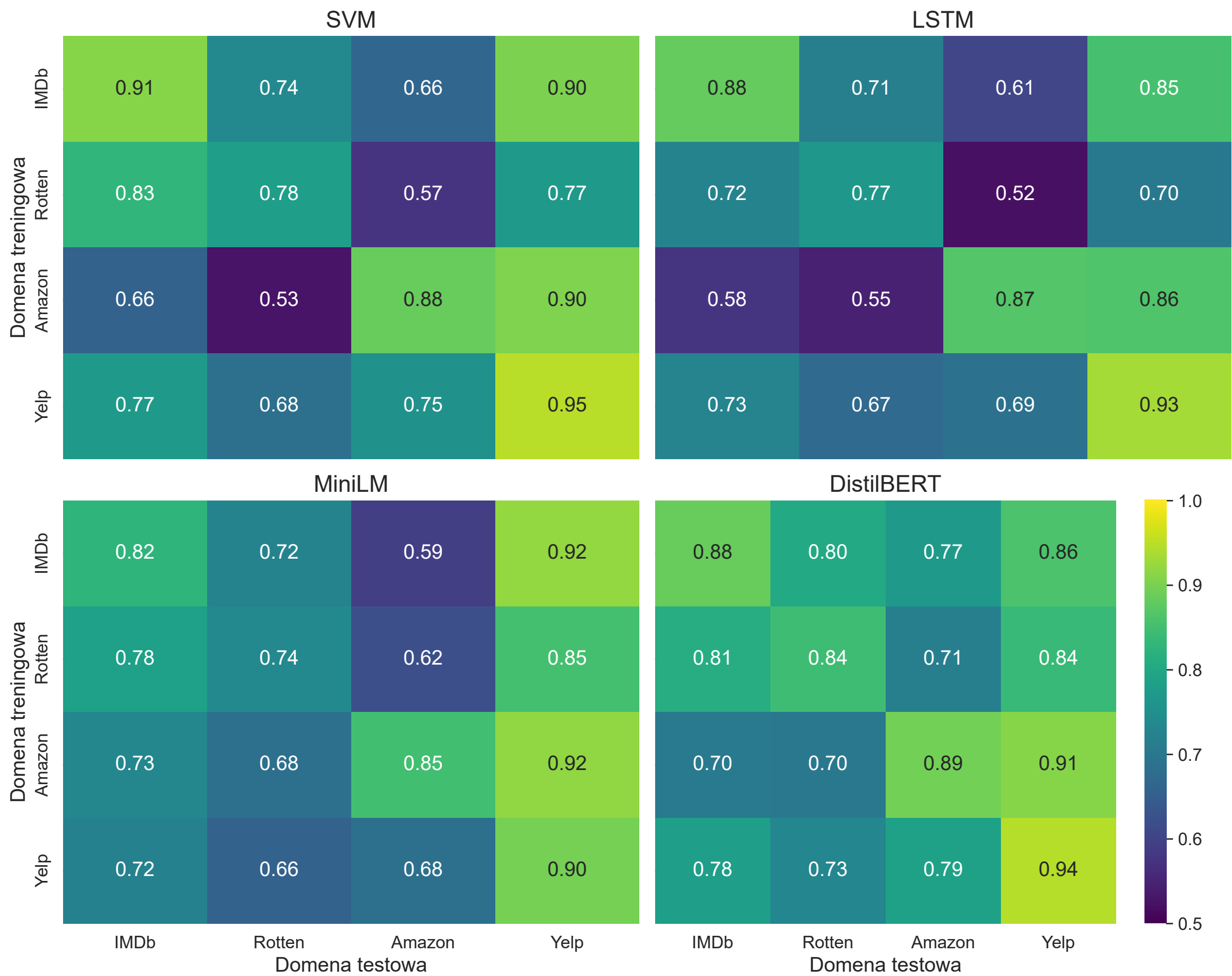
Średnie F1 (5 foldów) w macierzy cross-domain
