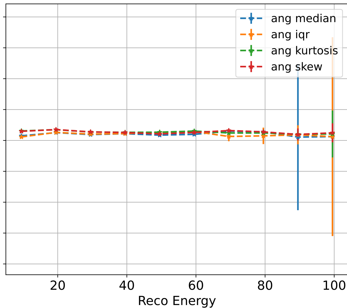
EM vs Hadronic Showers
