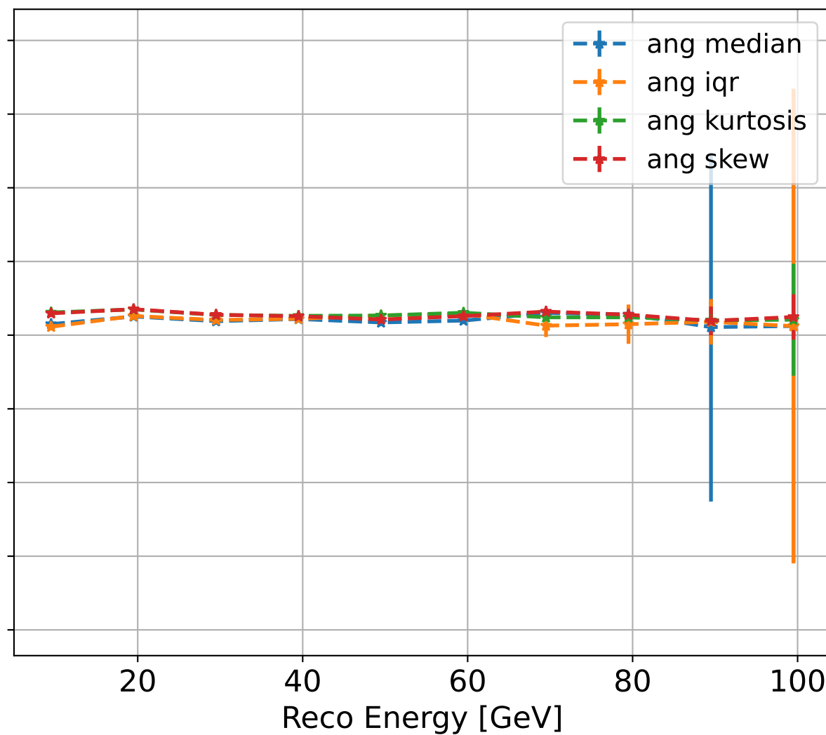
EM vs Hadronic Shower
