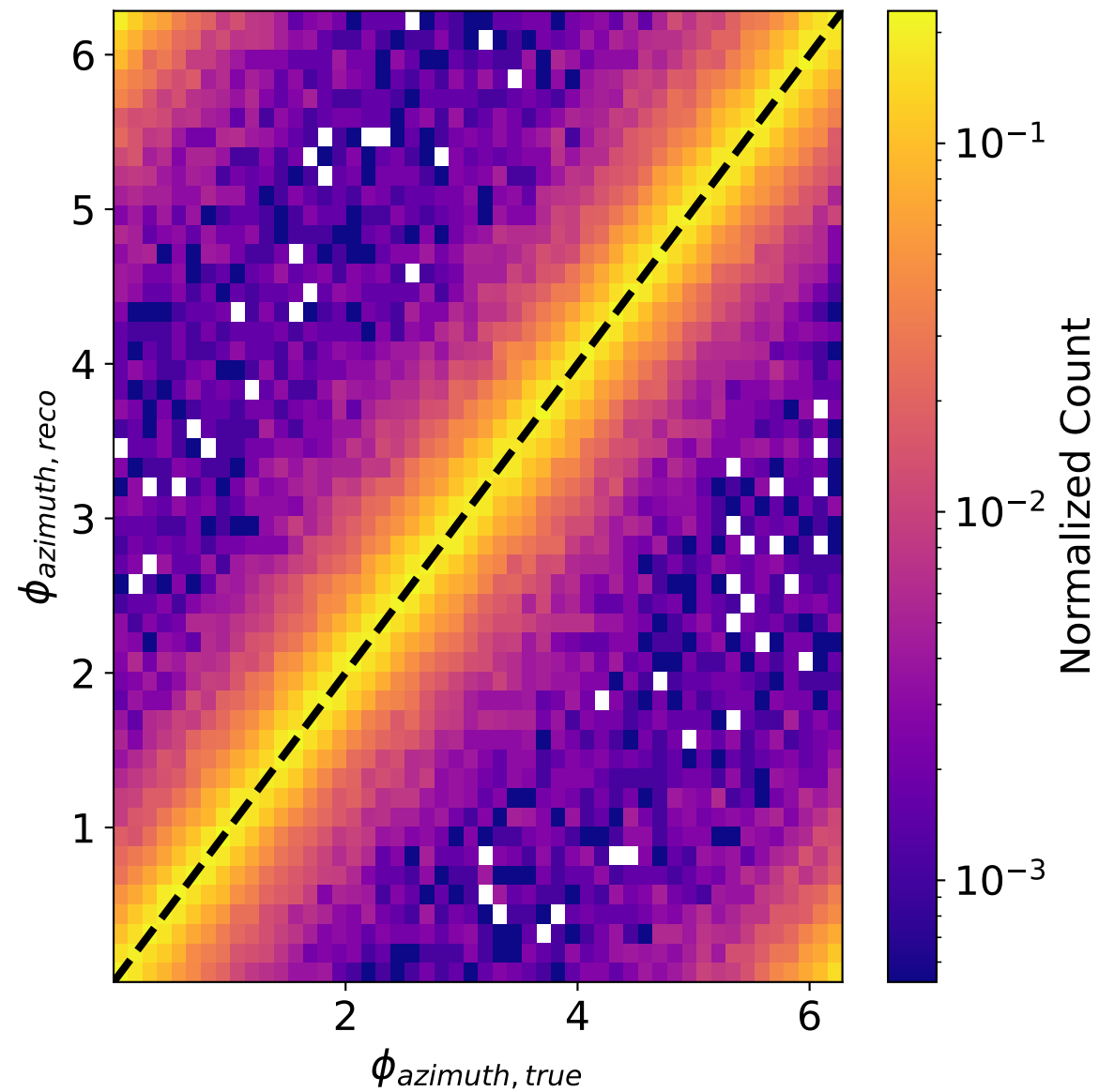
EM
