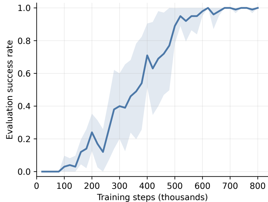
DDQN
