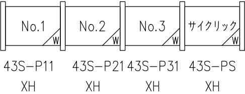
汚水ポンプ先発号機切替SW
