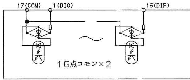
回路構成
