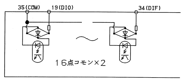
回路構成
