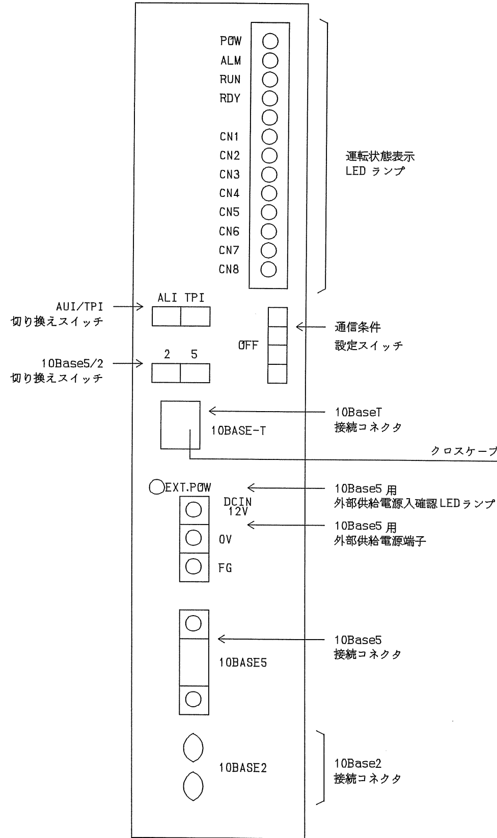
前面図
