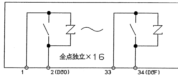
回路構成
