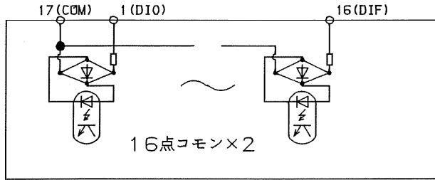
回路構成
