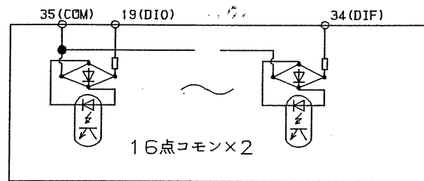
回路構成
