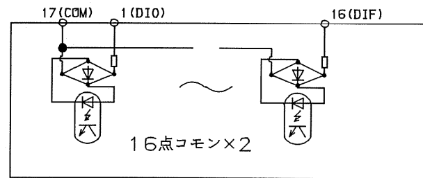
回路構成
