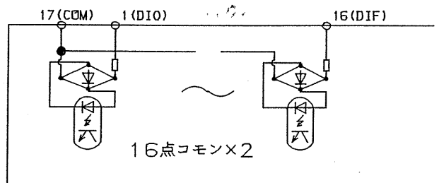
回路構成
