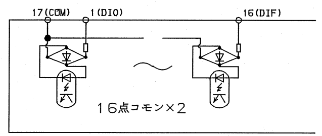
回路構成
