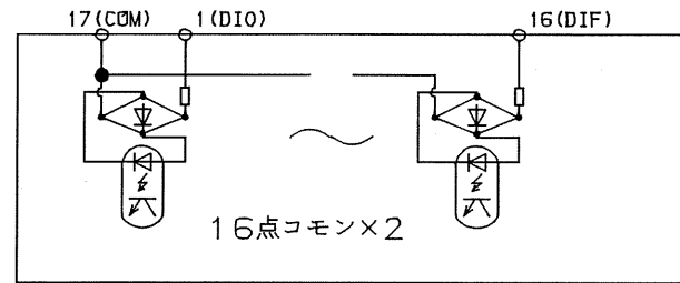
回路構成
