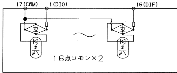
回路構成
