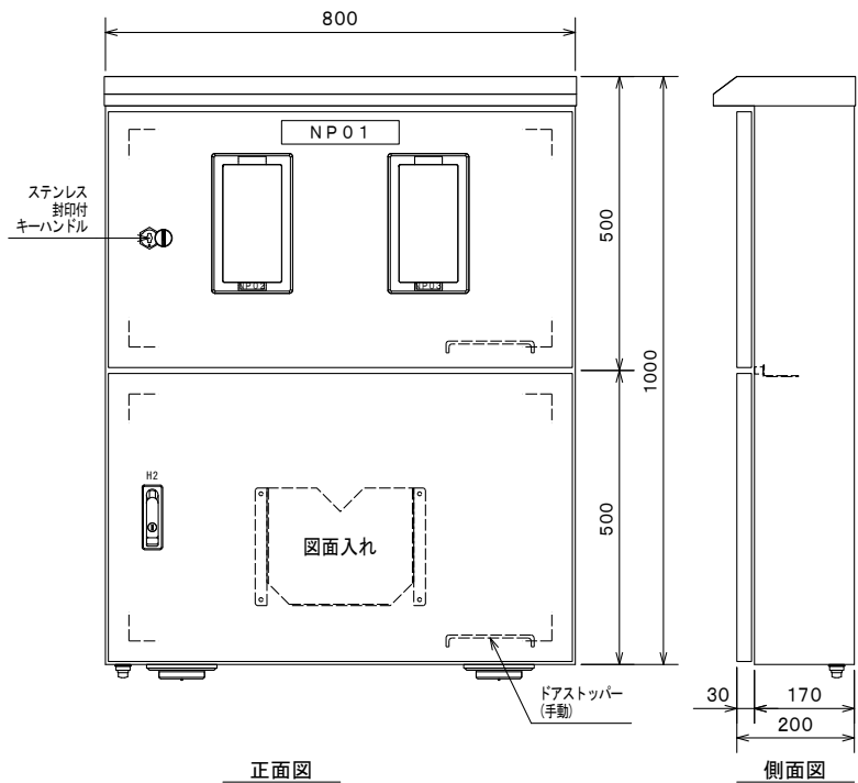
正面図
