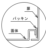
扉部構造図
