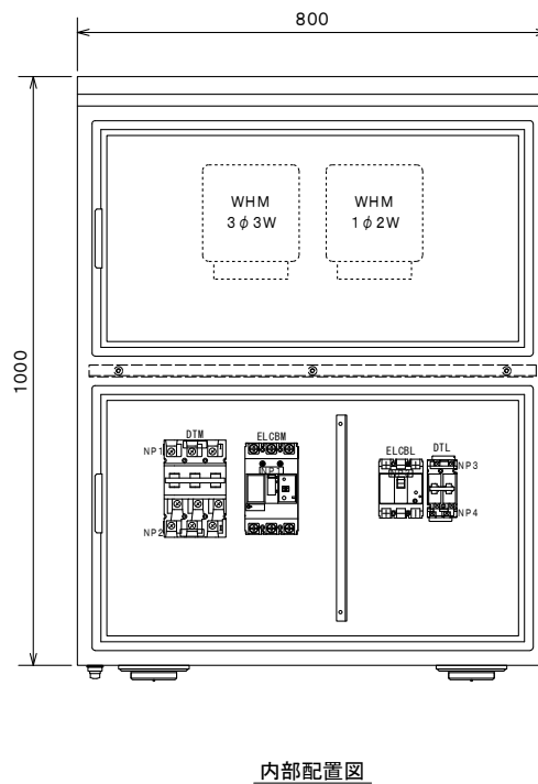
内部配置図
